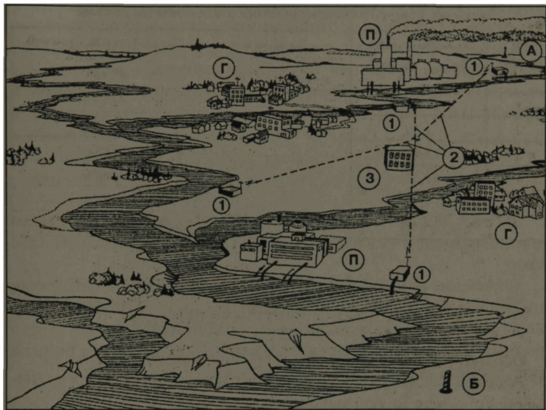
Рис. 1.7. Схема размещения элементов системы контроля качества воды на участке реки: А и Б – граничные створы системы; Г – населенные пункты; П – предприятия; 1 – места взятия проб воды, 2 – каналы связи; 3 – центр регистрации и обработки данных
