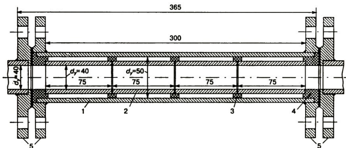
Рис. 1.3. Трубчатый индикатор коррозии и накипеобразования: 1 — корпус-патрон; 2 — индикатор; 3 — резиновые прокладки между индикаторами; 4 — то же между концами индикаторов и патроном; 5 — фланцы
