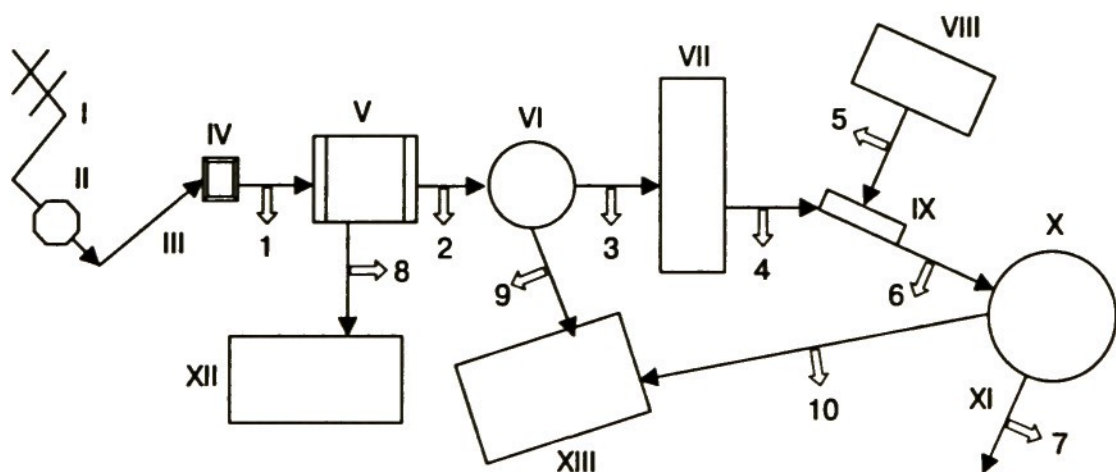
Рис. 2.3. Схема сооружений биологической очистки сточных вод в искусственно созданных условиях с указанием мест взятия проб (1–10) для лабораторного контроля:
