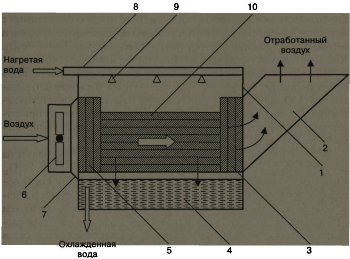
Рис. 1.10. Схема поперечно-точной градирни с сетчатым оросителем: 1 — корпус; 2 — воздухоотводящий раструб; 3 — водоуловитель; 4 — резервуар охлажденной воды; 5 — воздухораспределительное устройство; 6 — вентилятор; 7 — раструб; 8 — водораспределитель; 9 — форсунки; 10 — ороситель
