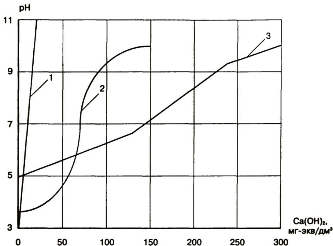
Рис. 2.10. Кривые титрования сточных вод завода химических реактивов: 1 — проба воды со слабо выраженными буферными свойствами; 2 — то же со средней буферностью; 3 — то же с сильной буферностью
