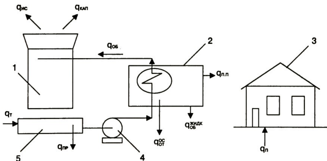
Рис. 1.4. Схема охлаждающей системы оборотного водоснабжения промышленного предприятия: 1 — градирня; 2 — теплообменная аппаратура промышленного предприятия; 3 — потребители питьевой воды на промплощадке; 4 — циркуляционный насос; 5 — водосборный бассейн градирни
