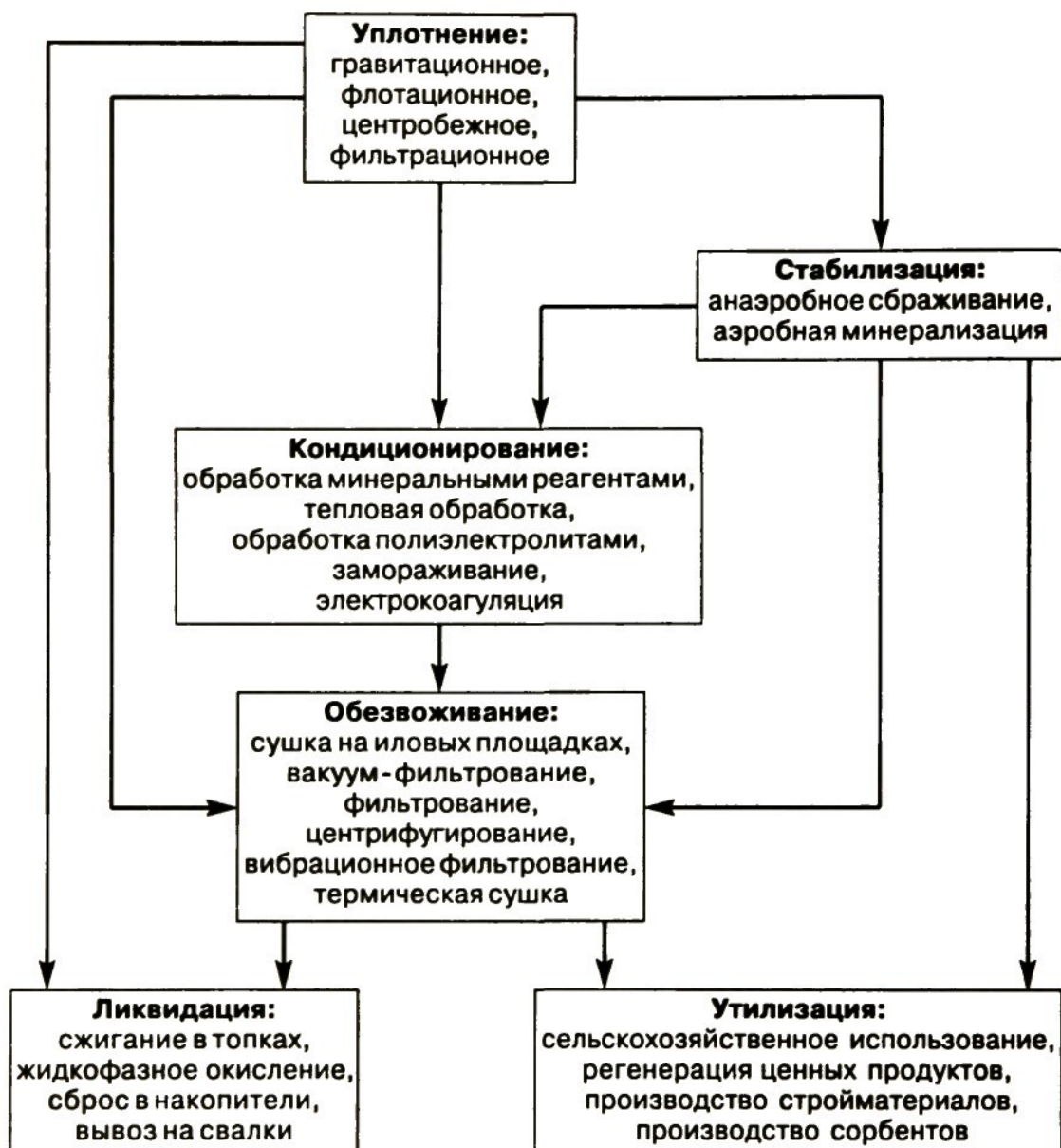
Рис. 2.7. Типовые процессы, применяемые для обработки осадков сточных вод
