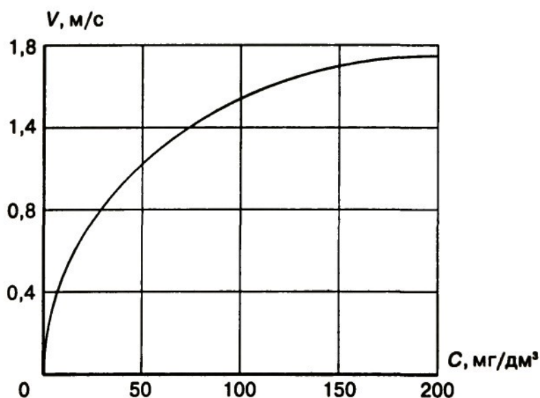
Рис. 1.5. Зависимость допустимой скорости движения оборотной воды в трубках теплообменных аппаратов (V) от концентрации взвешенных веществ в ней (C)
