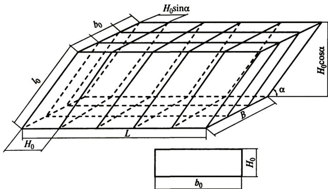
Рис. 1.8. Конструктивные параметры тонкослойных элементов в блоке:
