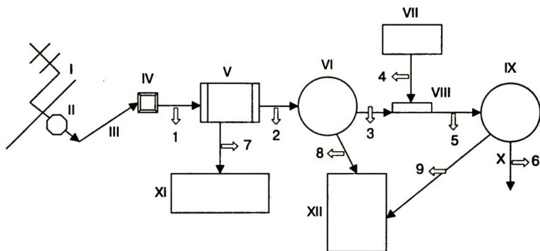
Рис. 2.2. Схема сооружений механической очистки сточных вод в естественных условиях с указанием мест взятия проб (1–9) для лабораторного контроля:
