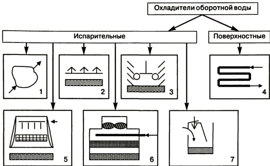
Рис. 1.6. Классификация охладителей оборотной воды: 1 – водохранилище (пруд-охладитель); 2 – брызгальный бассейн; 3 – открытые градирни; 4 – радиаторные градирни; 5 – башенные градирни; 6 – вентиляторные градирни; 7 – эжекционные градирни
