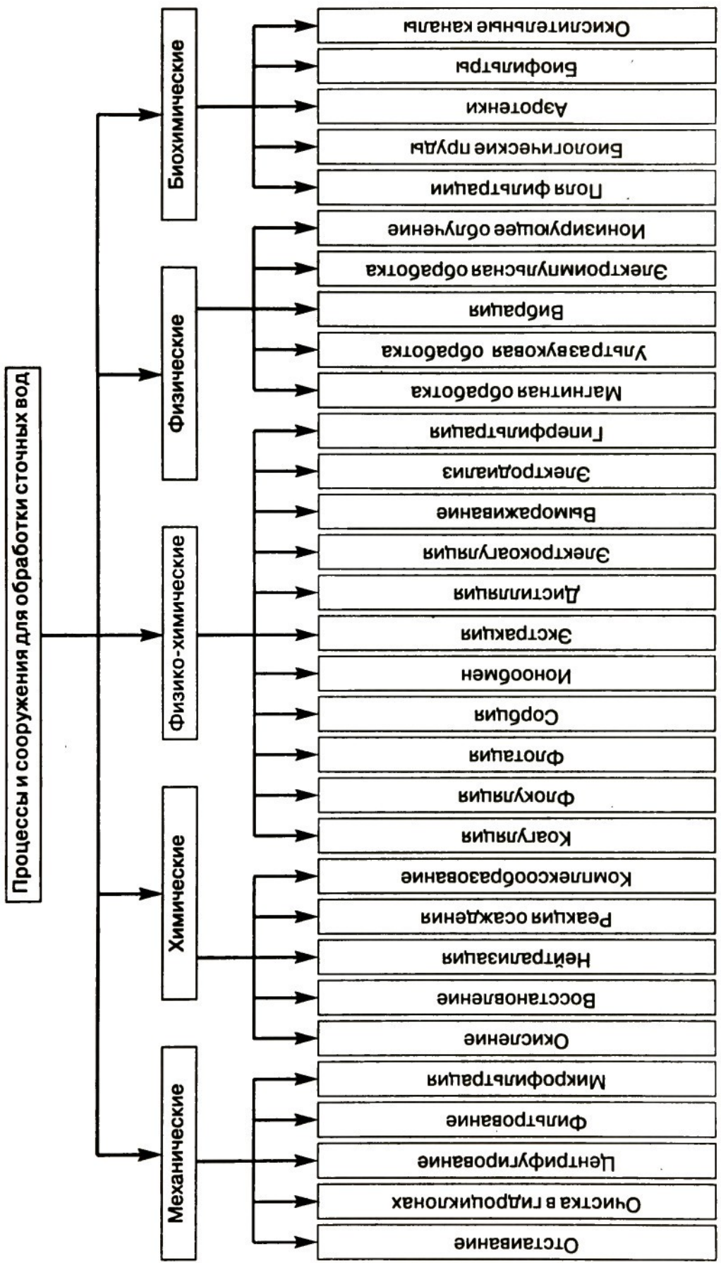
Рис. 2.5. Классификация процессов и сооружений для обработки сточных вод
