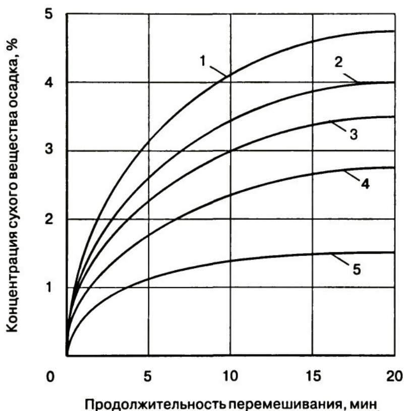
Рис. 2.8. Влияние продолжительности и скорости перемешивания на степень сгущения осадка:
