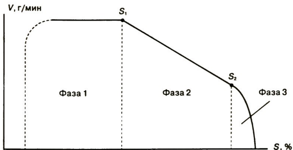
Рис. 2.6. Кривая обезвоживания осадка выпариванием при постоянной температуре. Здесь V — скорость сушки; S — содержание сухого вещества в образце, %; S_1 и S_2 — соответственно первая и вторая критические точки
