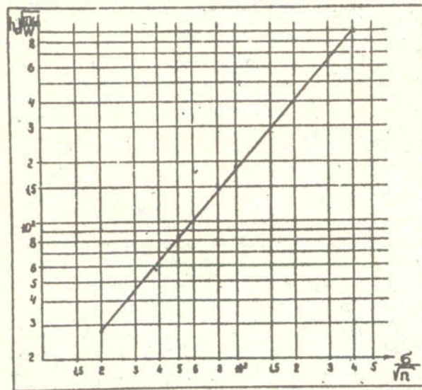
Рис. 4.1б. График зависимости h_r \sqrt{\frac{4K_1}{W}} = f\left(\frac{\sigma}{\sqrt{n}}\right)
