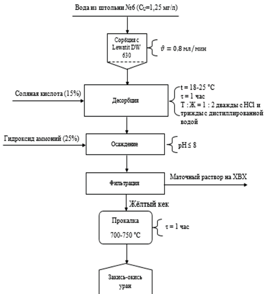
Рисунок 1. Принципиальная новая технологическая схема процесса очистки воды штольни №6 от радиоактивных и тяжелых металлов.
