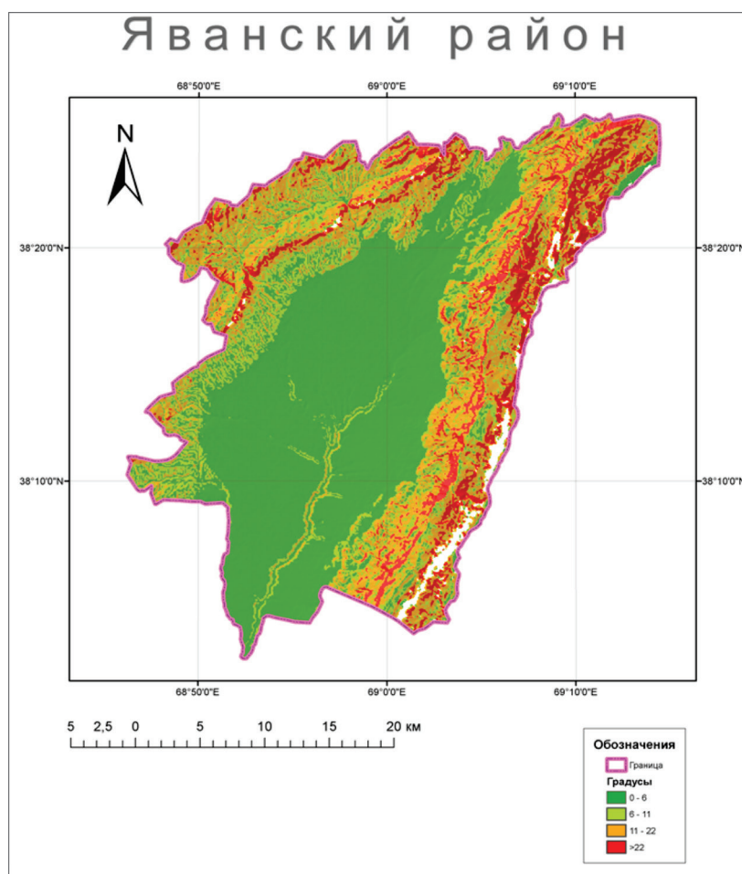
Рисунок 2. Карта уклонов.
