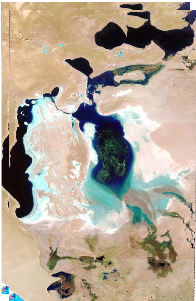
Космический снимок Landsat 8 2 Апрель 2018 год
