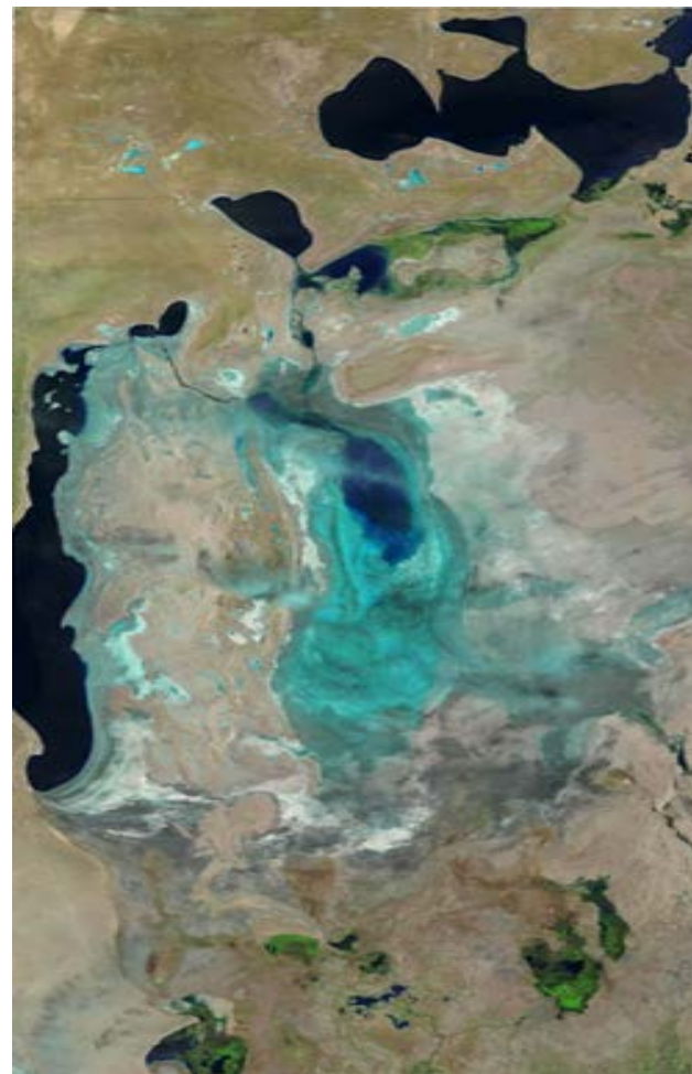
Космический снимок Landsat 8 7 Май 2019 год
