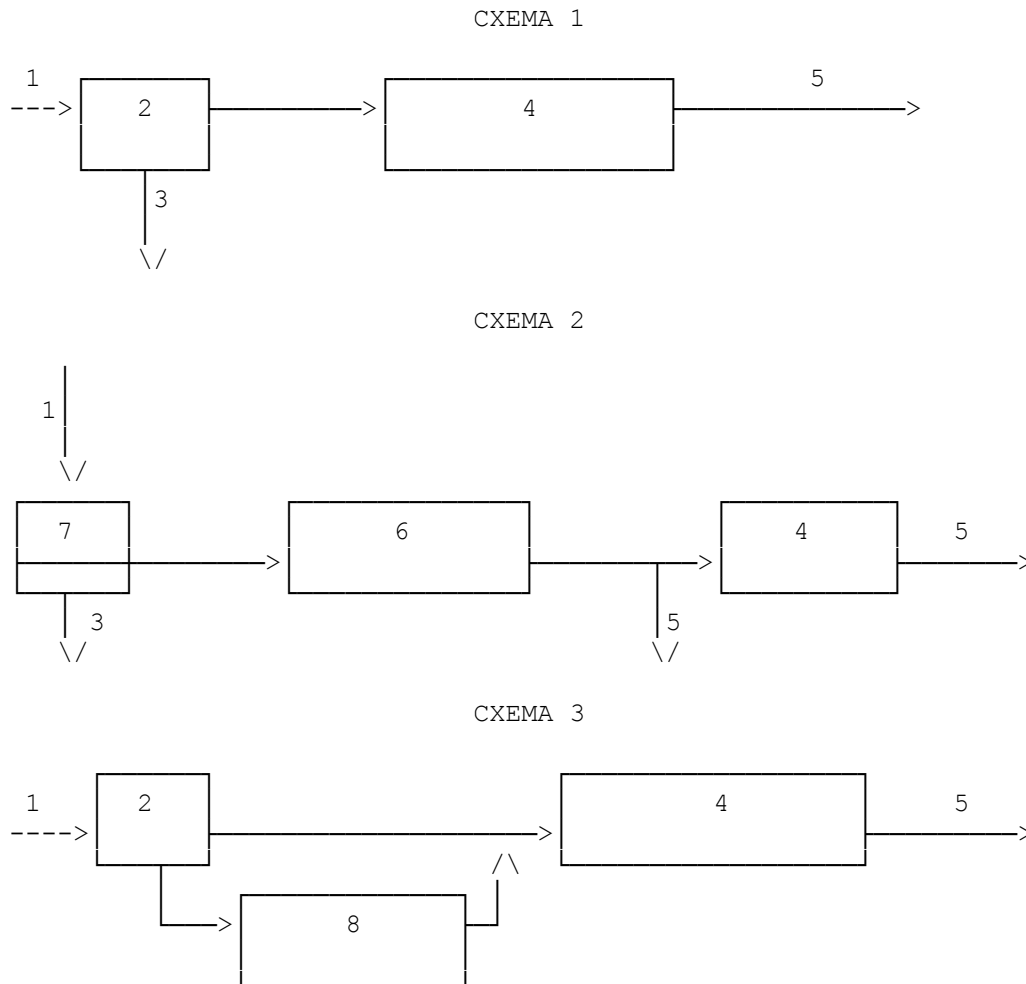
Рис. 1. Принципиальные схемы разделения дождевого стока перед очистными сооружениями:
