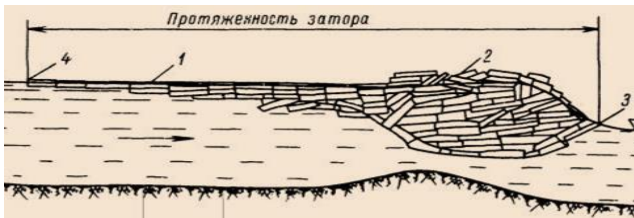
Рис. 3.1. Продольный разрез затора льда на реке.
