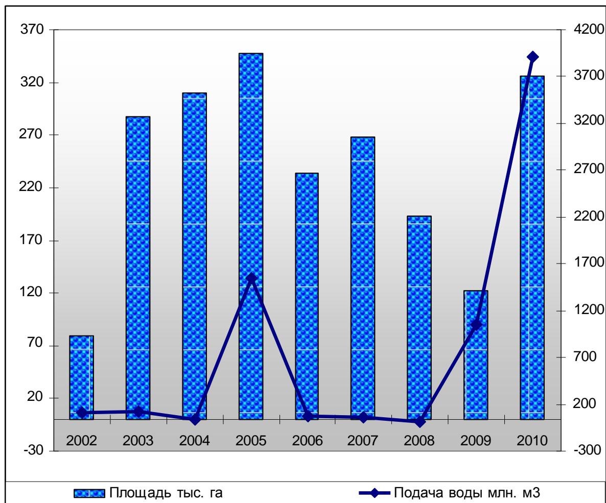
Рис. Динамика изменения площади ветландов в августе и подача воды в дельту реки Амударьи-г/п Саманбай
