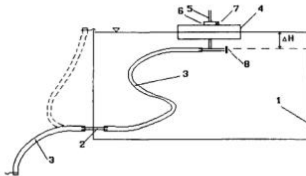
1 - емкость вместимостью 0,2 м 3 ; 2 - патрубок; 3 - резиновый шланг; 4 - поплавок из пенопласта; 5 - воздушная трубка; 6, 7 - регулировочный винт; 8 - сменная шайба с калиброванным отверстием; 9 - уровень воды в емкости
