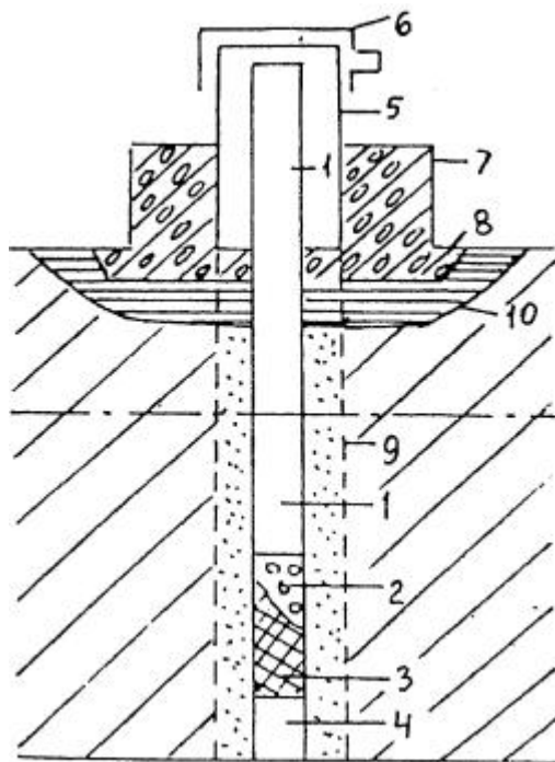
Рис. 3. Конструкция наблюдательной скважины:
