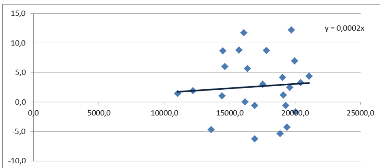
Рис. 31. Зависимость невязки руслового баланса на участке Келиф – Бир-Ата (Y, %) от стока Амударьи в створе Келиф (X, млн. м 3 ) за октябрь–март (по данным 1991-2017 гг.)
