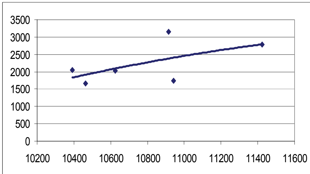
Рис. 16. Эмпирическая связь годового количества потерянной электроэнергии на холостых сбросах (ось Y) от используемого количества электроэнергии, вырабатываемой на Нурекской ГЭС (ось X)
