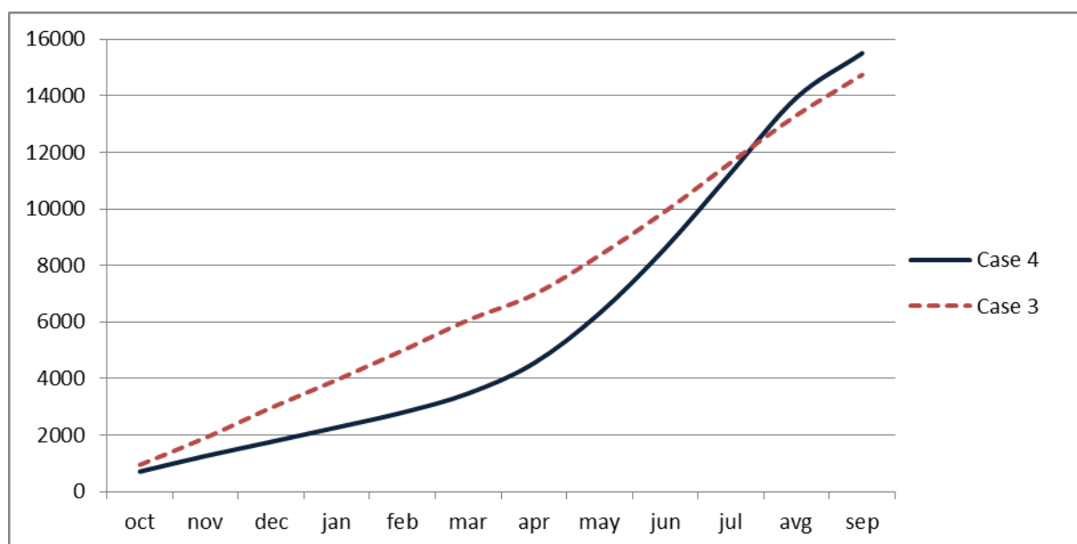
Рис. 107 Интегральная кривая месячной выработки э/э на Вахшском каскаде ГЭС (включая Нурекскую ГЭС): осреднение за 2020-2055 гг, при энергетическом (case 3) и энерго-ирригационном (case 4) режимах работы Нурекской ГЭС, млн.кВт.ч
