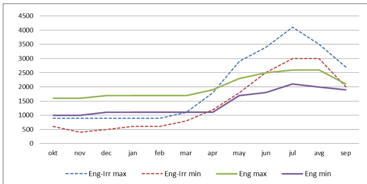
Рис. 18. Диапазон попусков из Нурекского г/у для энергетического и энерго-ирригационного режимов работы ГЭС, млн.м 3 /мес
