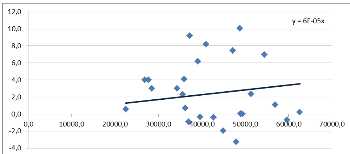
Рис. 32. Зависимость невязки руслового баланса на участке Келиф – Бир-Ата (Y, %) от стока Амударьи в створе Келиф (X, млн. м 3 ) за апрель–сентябрь (по данным 1991-2017 гг.)
