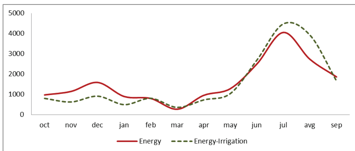
Рис. 45 Гидрограф стока реки Амударья в створе г/п Бирата (приток к ТМГУ) для особо маловодного года (2042-2043 г) для вариантов: case 1 (энергетический) и case 2 (энерго-ирригационный), млн.м 3 /мес
