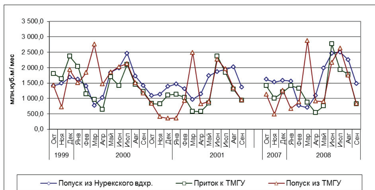
Рис 92 Попуски из Нурекского и Тюямуонского водохранилищ в маловодные годы
