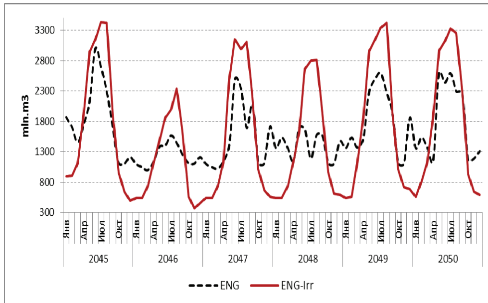
Рис. 23. Пример отображения информации. Попуски из Нурекского ГЭС при энергетическом (Eng) и энерго –иригационном (Eng-Irr) режимах: выборка из БД для периода 2045-2050 гг.
