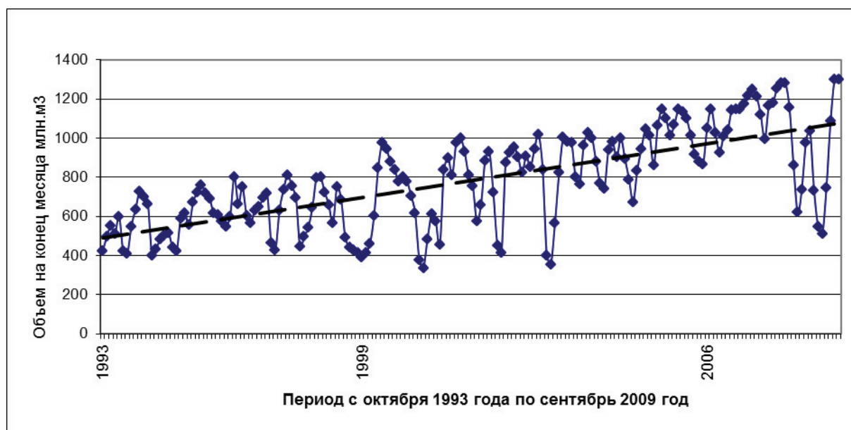
Рис. 94. Динамика объемов воды в Зейдском водохранилище
