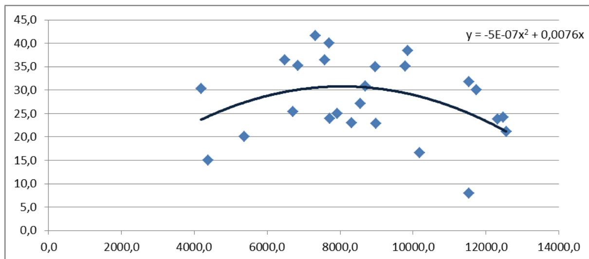
Рис. 33. Зависимость невязки руслового баланса на участке Тюямуюн–Саманбай (Y, %) от стока Амударьи ниже ТМГУ (X, млн. м 3 ) за октябрь–март (по данным 1991-2017 гг.)
