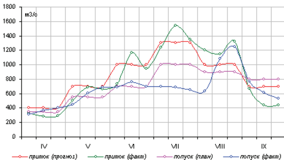
Рис 5. Притоки и попуски Нурекского водохранилища в маловодную вегетацию 1995
