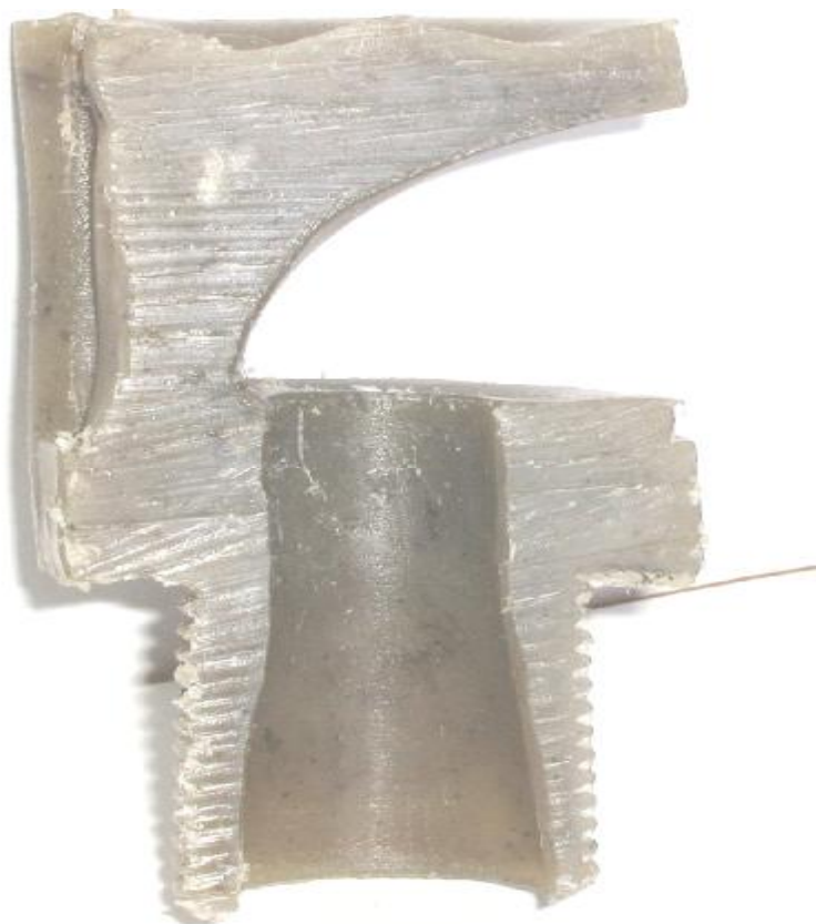
Рис. 6. Секторный насадок в разрезе
