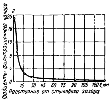
Рис. 41. Изменение градиентов фильтрационного напора вдоль керамической трубки (ширина зазора между трубками \tau = 1,1 мм, напор над дреной H = 37 см).
