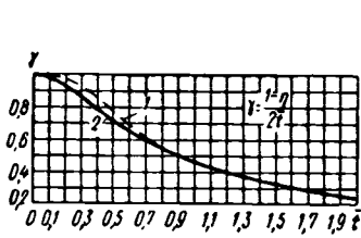
Рис. 31. Зависимость \bar{i}=f(\gamma) : 1 — при \eta=1 ; 2 — при \eta \geq 5 .
