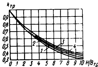
Рис. 14. Зависимость k_{\text{тр}} = f(H/B_{\text{тр}}) :
