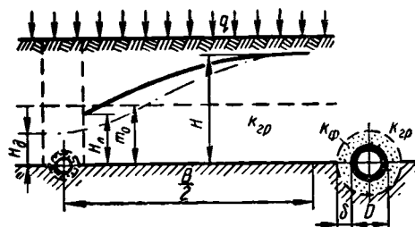
Рис. 22. Расчетная схема дрены на водоупоре.
