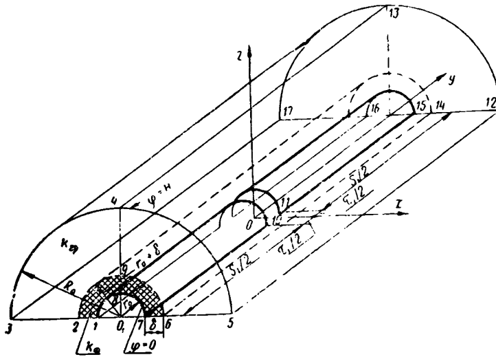
Рис. 7. Расчетная область фильтрации для керамического дренажа, уложенного с фильтром.
