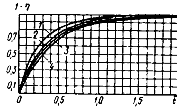
Рис. 32. Зависимость \bar{i}=f(\eta, \eta_m) : 1 — при \eta_m=0,5 ; 2 — при \eta_m=1 ; 3 — при \eta_m=2 ; 4 — при \eta_m \geq 3 (по С. Ф. Аверьянову).
