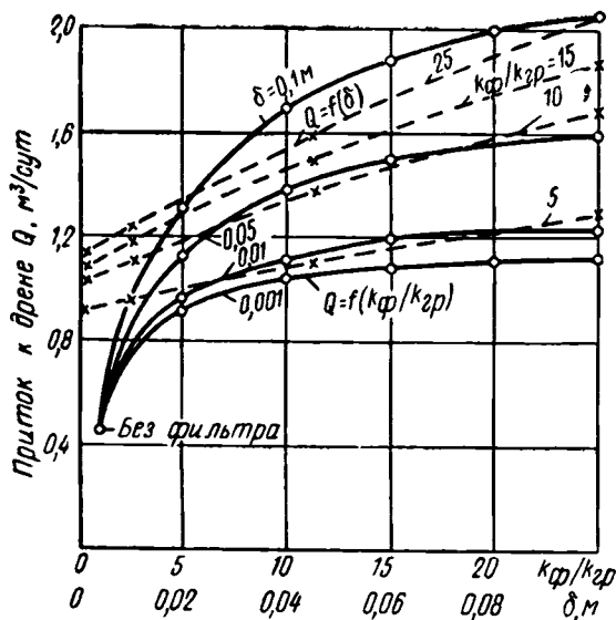
Рис. 50. Зависимости Q=f(k_{\phi}/k_{гр}, \delta=\text{const}) и Q=f(\delta, k_{\phi}/k_{гр}=\text{const}) для керамической дрены: S_1=0,33 м; \tau_1=0,002 м; r_0=0,036 м; k_{гр}=1 м/сут; H=0,5 м; R=0,5 м; L=1 м.
