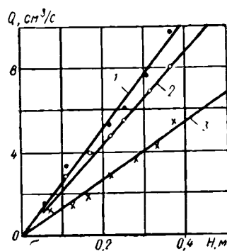
Рис. 48. Зависимость Q=f(H) для керамической дрены (один стыковой зазор \tau_1=2 мм): 1 — с фильтром из стеклохолста толщиной 1 мм; 2 — с фильтром из песчано-гравийной смеси толщиной 25 мм; 3 — без фильтра.
