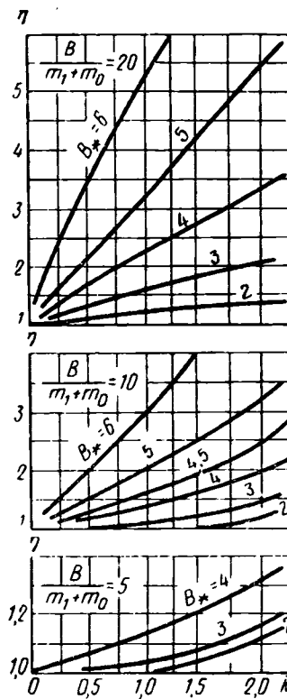
Рис. 30. Зависимость \eta = f(B/m_*, \bar{k}, B_*) .
