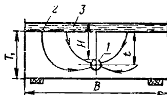
Рис. 52. Схема подрусловой дрены (лоток):
