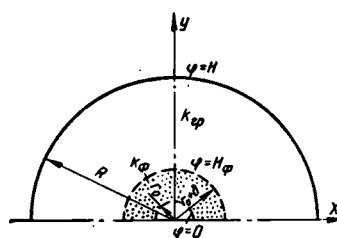
Рис. 6. Расчетная область фильтрации для трубофильтра.
