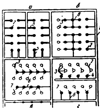
Рис. 61. Схемы систематического вертикального дренажа:
