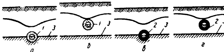
Рис. 4. Схема дрен:
