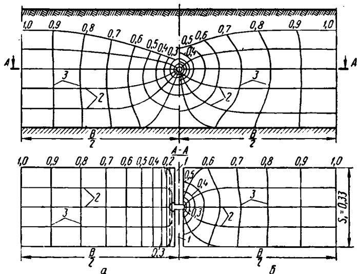
Рис. 46. Гидродинамическая сетка керамической дрены при боковом питании: а — с фильтром; б — без фильтра; 1 — керамическая трубка; 2 — линии тока; 3 — линии равных напоров.
