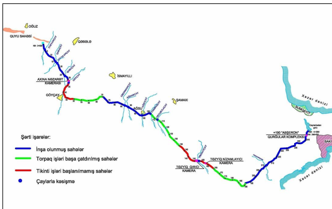
Рис. 9.1. План трассы водопровода Огуз-Габала-Баку
