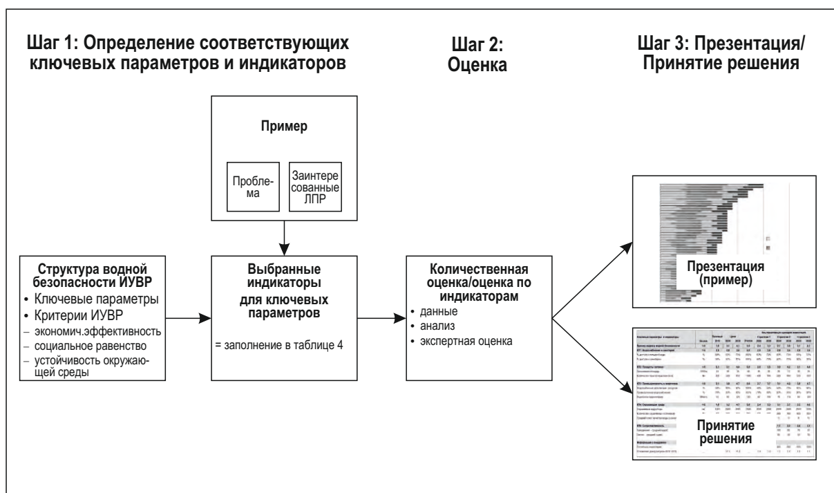
Рисунок 8. Три шага подхода развития к количественной оценке водной безопасности
