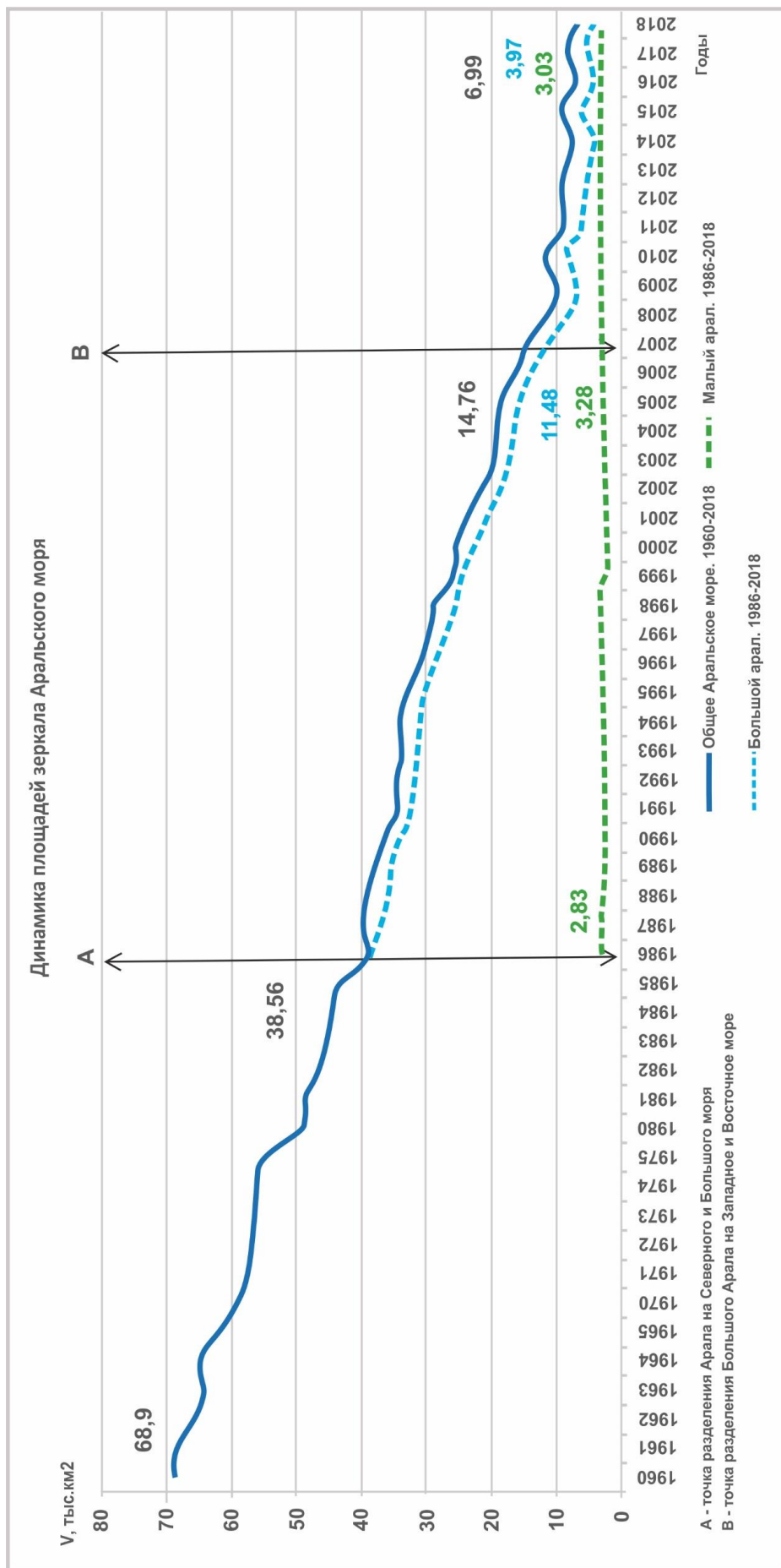
Рис. 2.2. Динамика площадей зеркала Аральского моря
