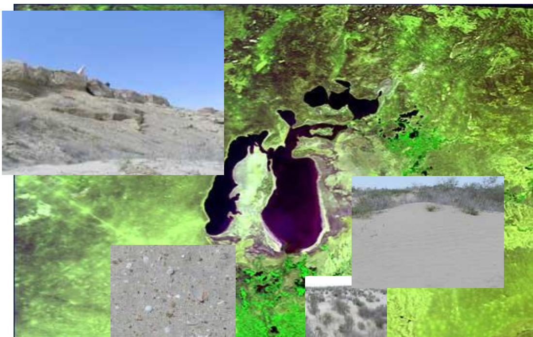
Рис. 4.2. Некоторые типы осушившегося побережья
