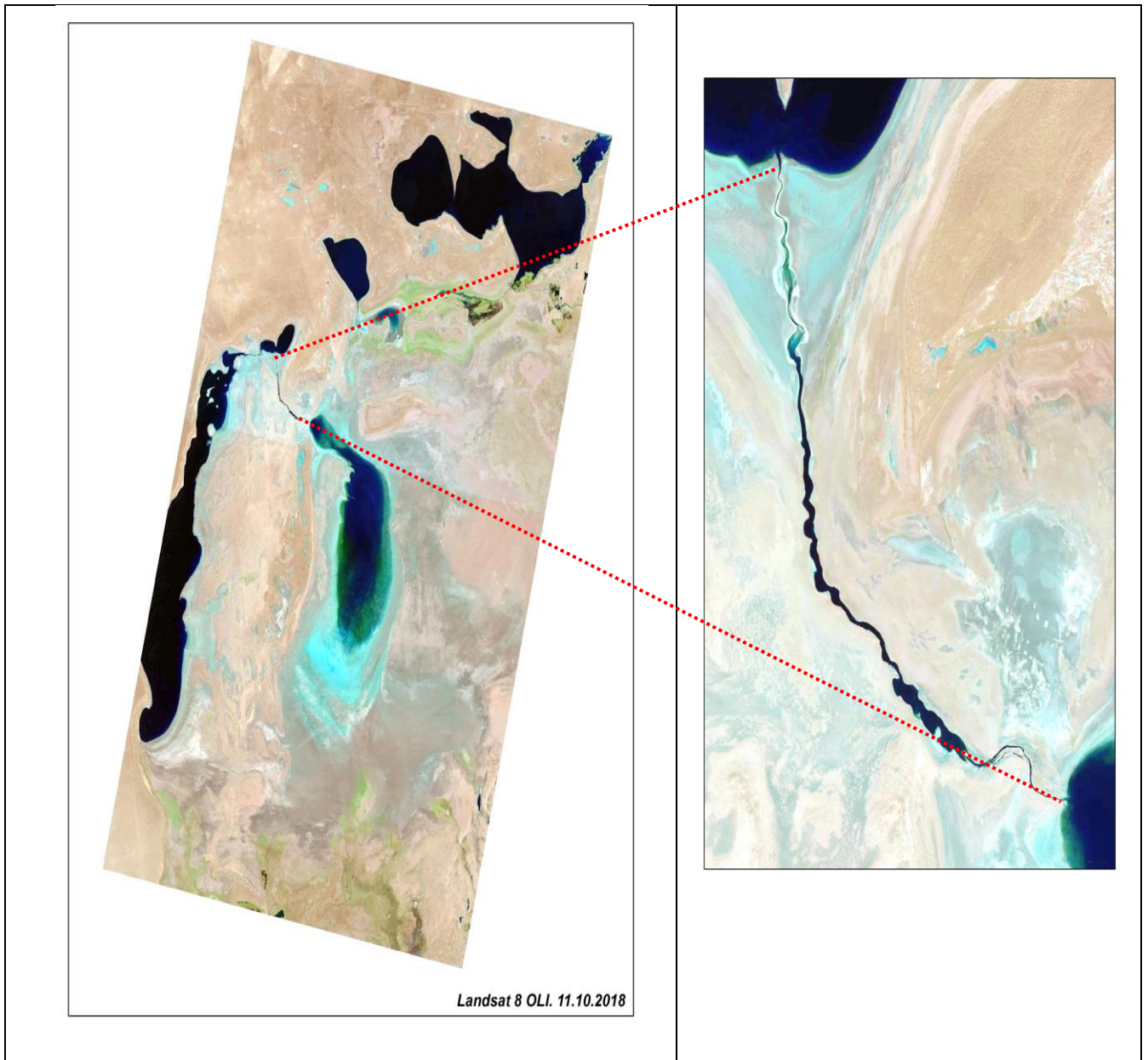
Рис. 2.12. Переток с Восточной части в Западную часть Большого Аральского моря
