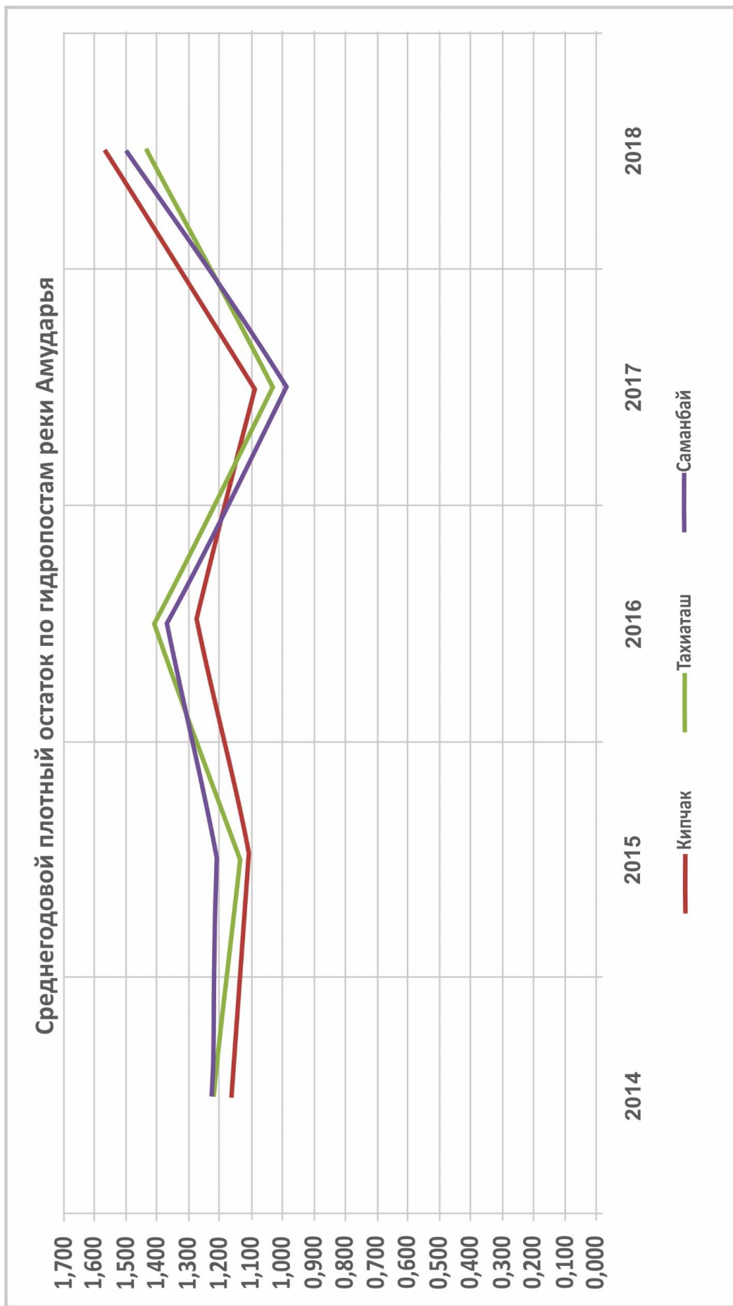
Рис.2.4. Средний годовой плотный остаток по гидропостам реки Амударья, г/л
