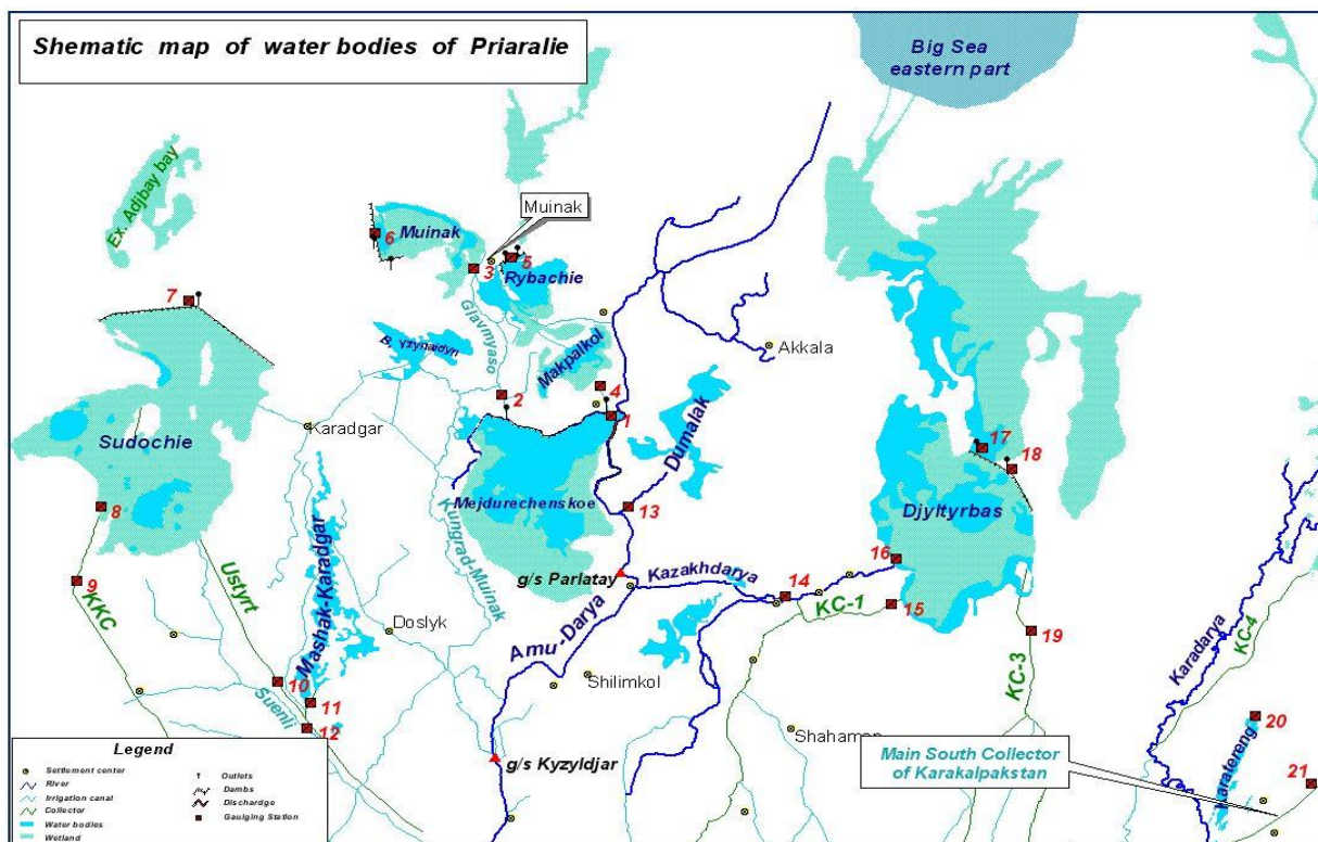
Рис.5.2. Схематическая карта расположения гидростов в зоне Приаралья (2011 г.)
