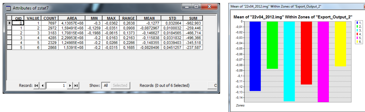
Рис. 8.6.1 Значения NDVI Landsat TM
