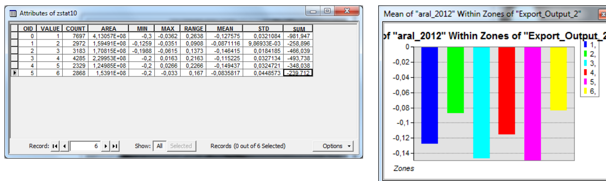
Рис. 8.6.2 Значения NDVI MODIS Terra
