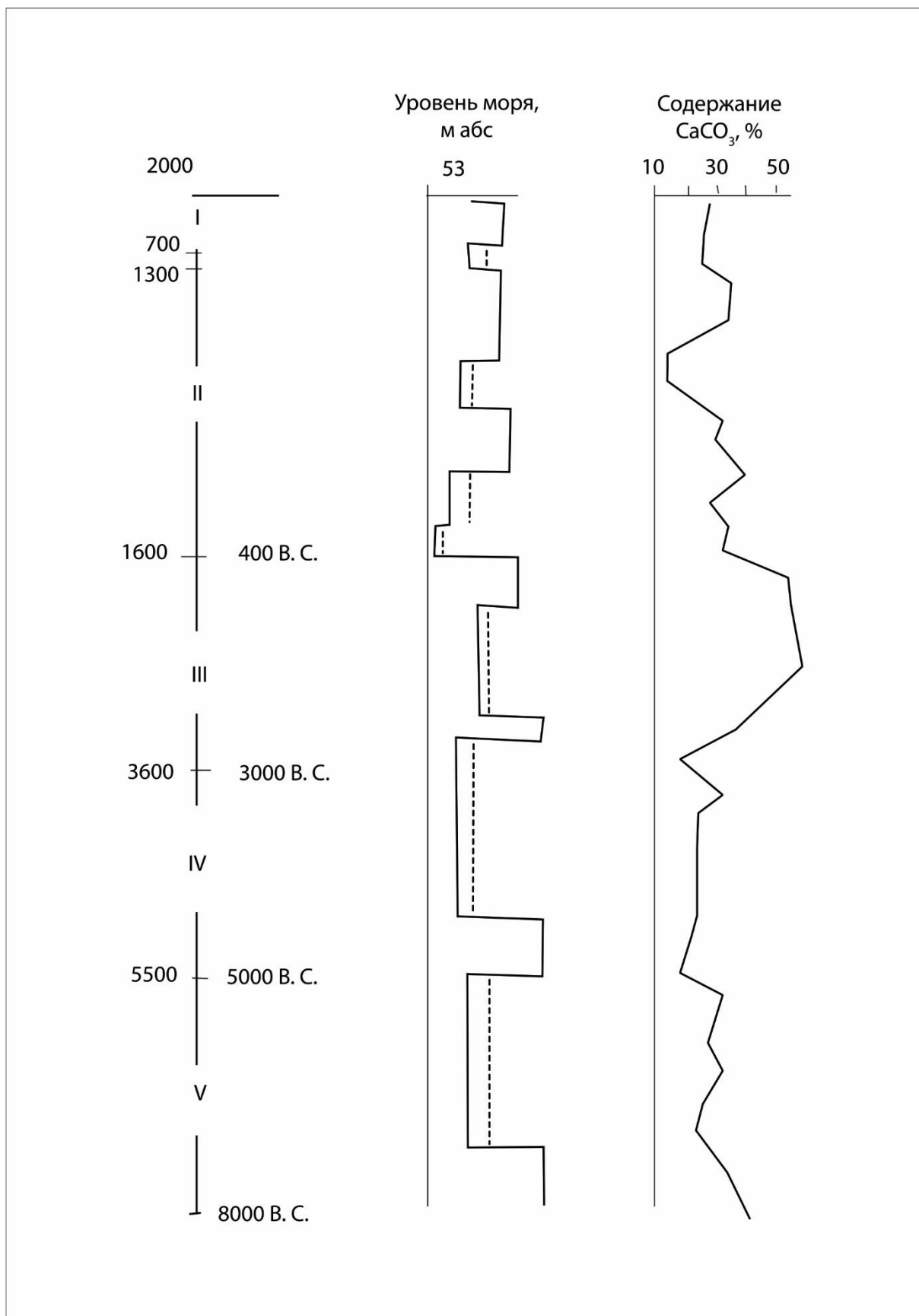
Рис. 1.2. Историческое развитие уровня моря и концентрация CaCO 3
