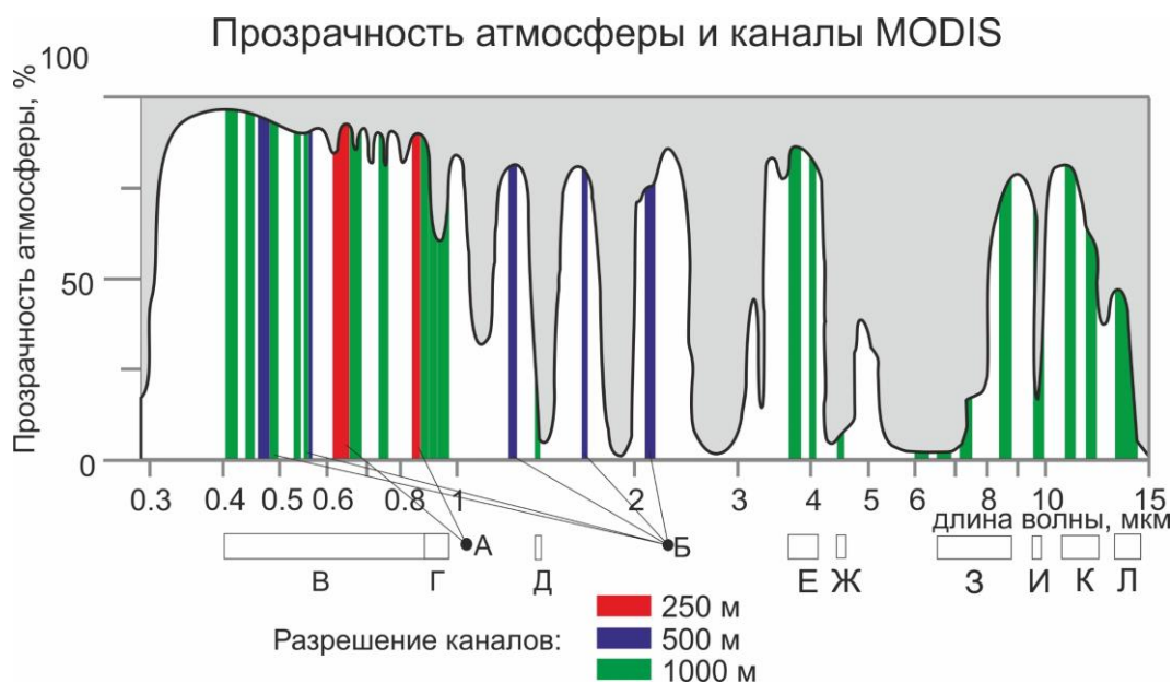
Рис. 8.4.1 Каналы космоснимка MODIS
