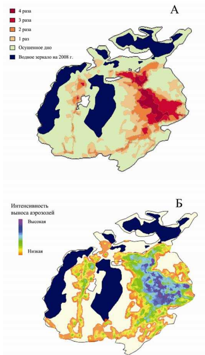
Рис. 6. Пространственные характеристики зон солепылевого выноса с осушенного дна Аральского моря в период 2005-2008 гг. А – частота попадания территории в зону солепылевого выноса при анализе годовых выборок за период 2005-2008 гг.
