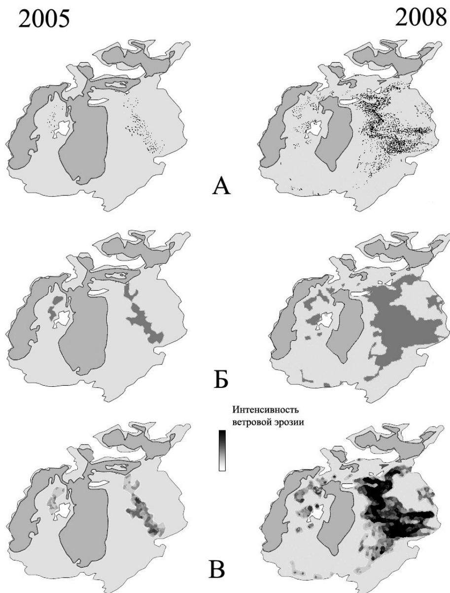
Рис. 5. Результаты спутникового мониторинга пыльных бурь с осушенного дна Аральского моря 2005 и 2008 годов: А – экспертная оценка интенсивности пыльных бурь на спутниковых сценах; Б – контуры зон солепылевого выноса (состояние водного зеркала дано по спутниковым данным на май рассматриваемого года); В – интенсивность процесса солепылевого выноса (усреднено за год)
