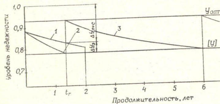
Рис. 4. Изменение уровня надежности дрены:
