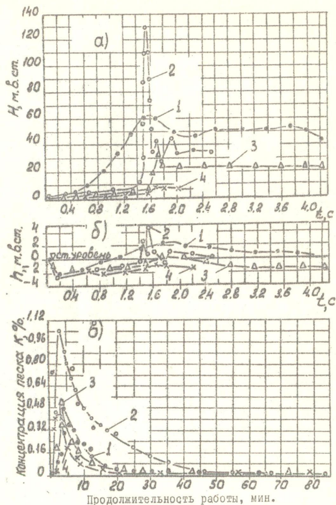
Рис. I. Зависимость переходных процессов в системе "насосная установка-скважина" от способа пуска насоса (ЭЦВ12-255-30М).
