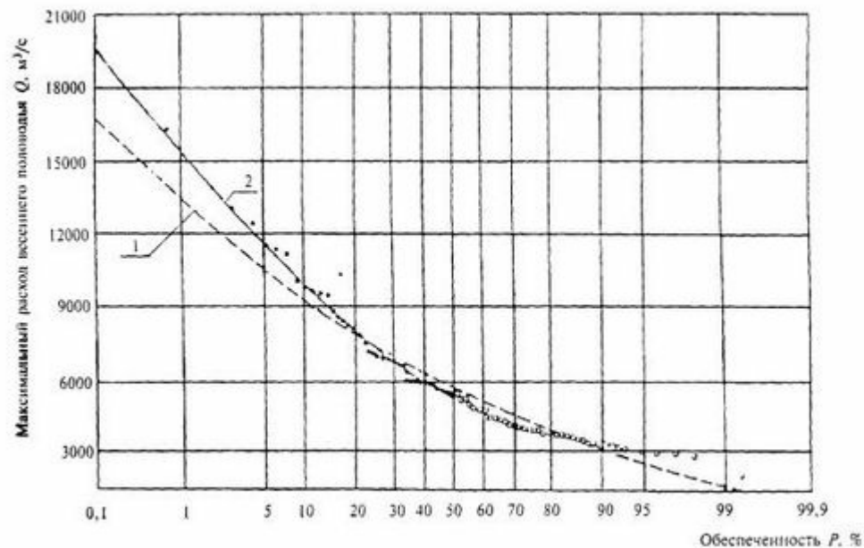
Гамма-распределение: 1 - полное; 2 - усеченное
