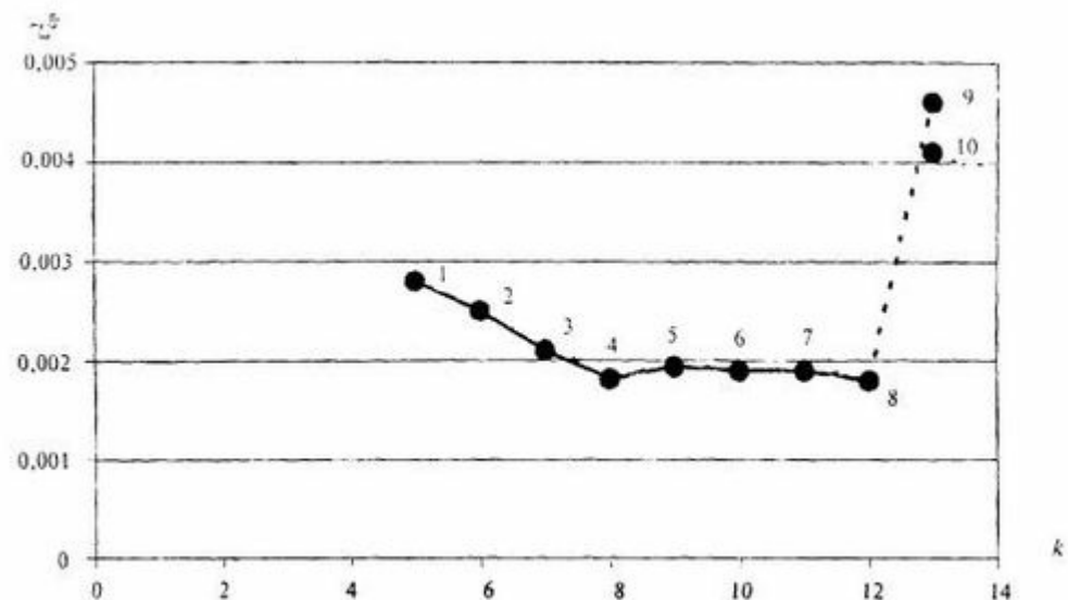
Рисунок А.3 - График зависимости дисперсии параметров объединенной совокупности от числа совместно анализируемых постов
