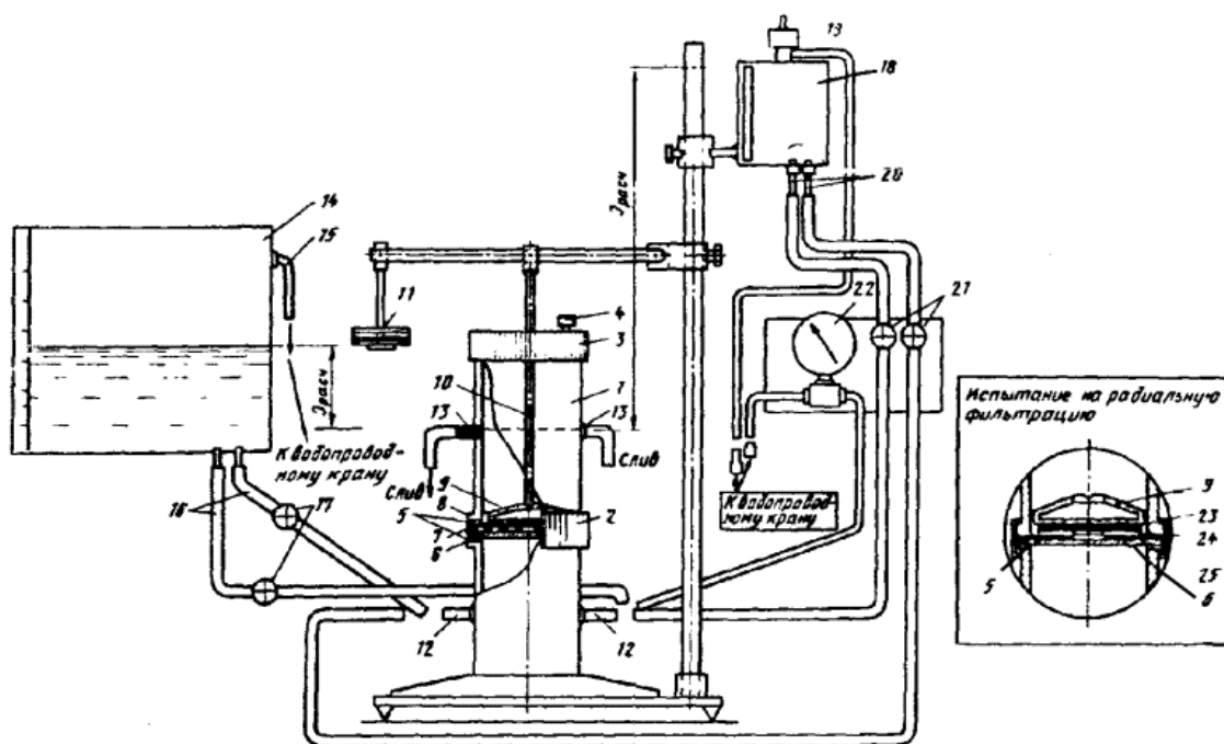
Рис. 1. Схема фильтрационного прибора:
