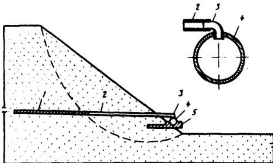
Рис. 9. Сброс грунтовых вод по коллектору:
