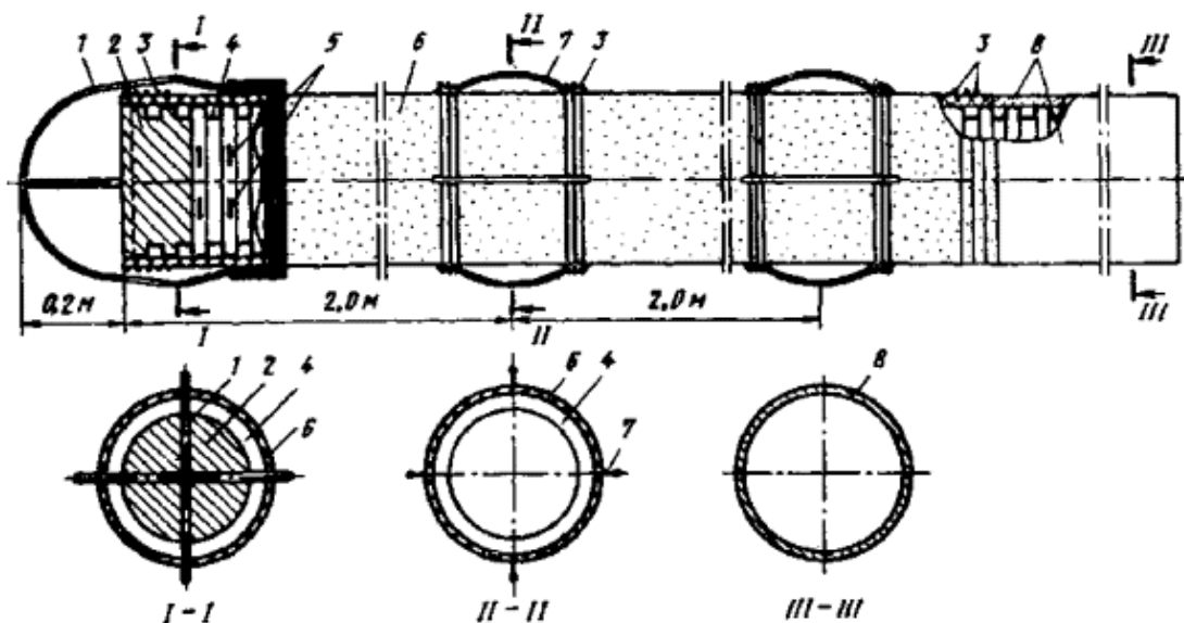
Рис. 10. Конструкция дрены:
