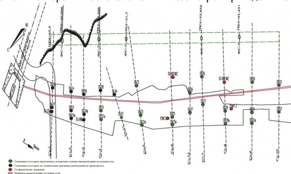
Рис. 1. План расположения пьезометрических скважин на участке левого берега солевого пласта р. Вахш
