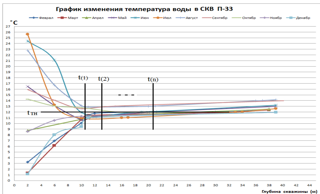
Рис. 2. График изменения температуры воды в П-33
