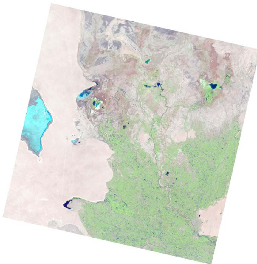
Рис. 2 Южное Приаралье. На основе снимка Landsat 8- 9. 23 сентября 2023
