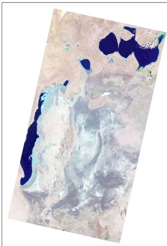
Рис. 1 Западное и Восточное Аральское море. На основе снимка Landsat 8 - 9. 23 сентября
