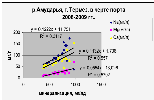
Рисунок 4.5 -Графики зависимости содержания главных ионов (Ca, Mg, Na, HCO 3 , Cl, SO 4 ) от величины минерализации р.Амударья – створ г.Термез
