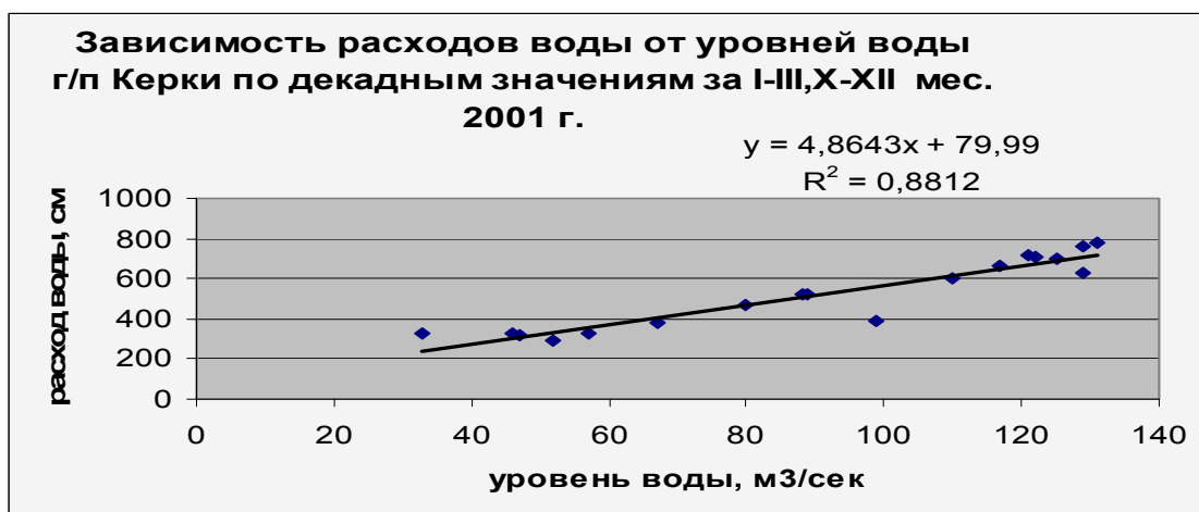
Рисунок 3.9- Зависимость расхода воды от уровня воды в створе Керки
