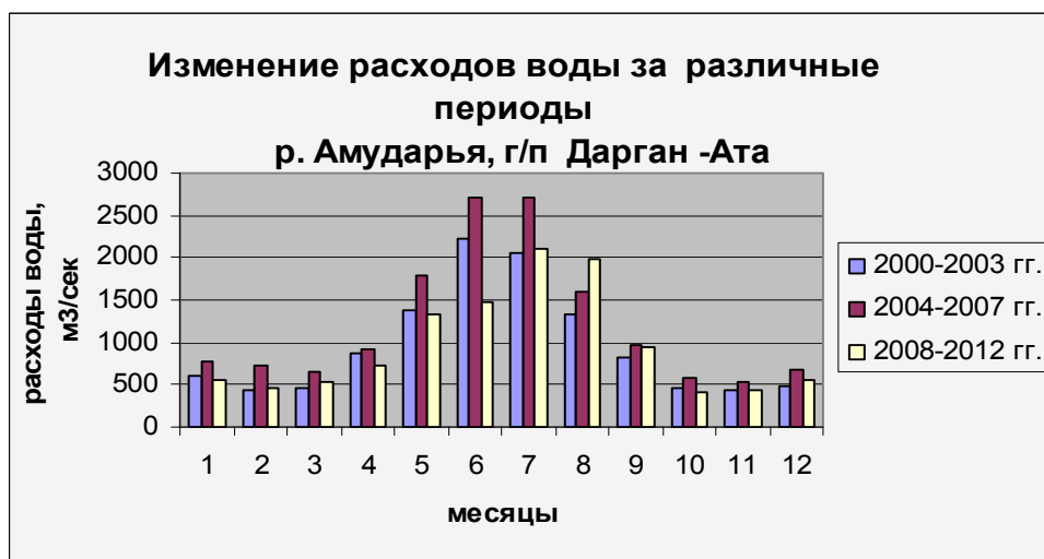
Рис. 3.7. - Анализ расходов воды р. Амударьи у г/п Дарганата за разные периоды
