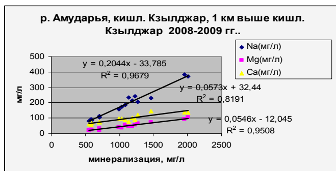
Рисунок 4.6 -Графики зависимости содержания главных ионов (Ca, Mg, Na, HCO 3 , Cl, SO 4 ) от величины минерализации на различных створах р. Амударья.
