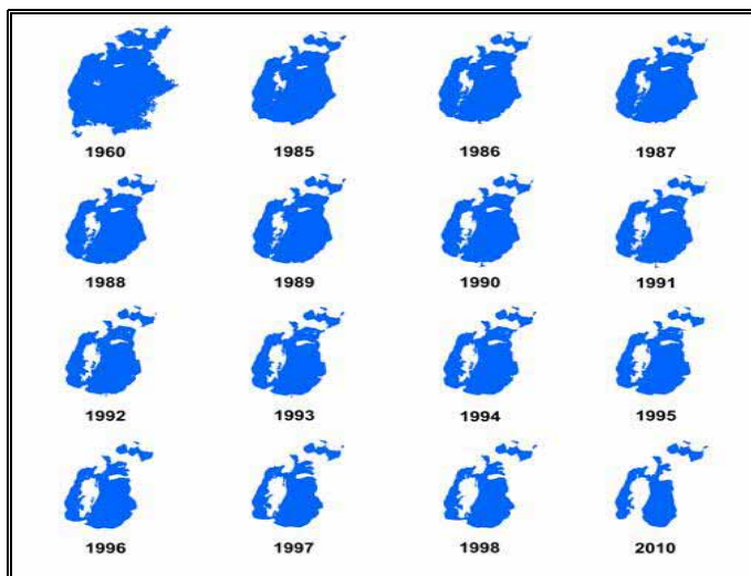
Рисунок 5.1-изменение уровня моря Аральского моря
