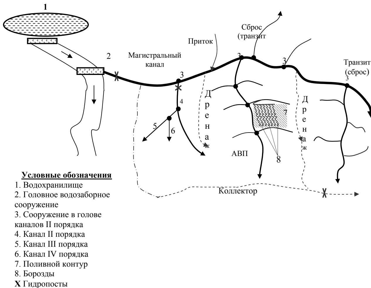
Рис. 2.1. Схема гидромелиоративной сети
