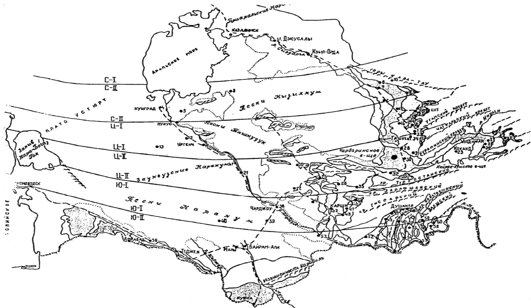
Рис. 1. Климатические зоны
