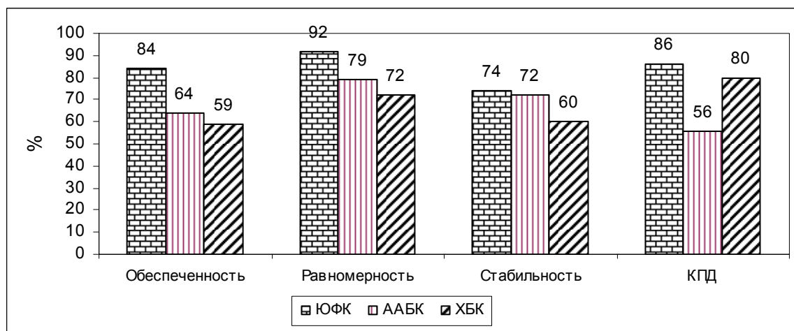
Рис. 1. Стабильность головного водозабора в ПК
