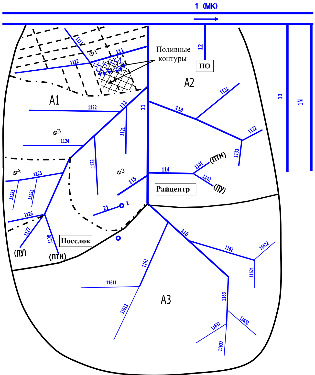
Рис. 2.2. Фрагмент схемы системы магистрального канала
