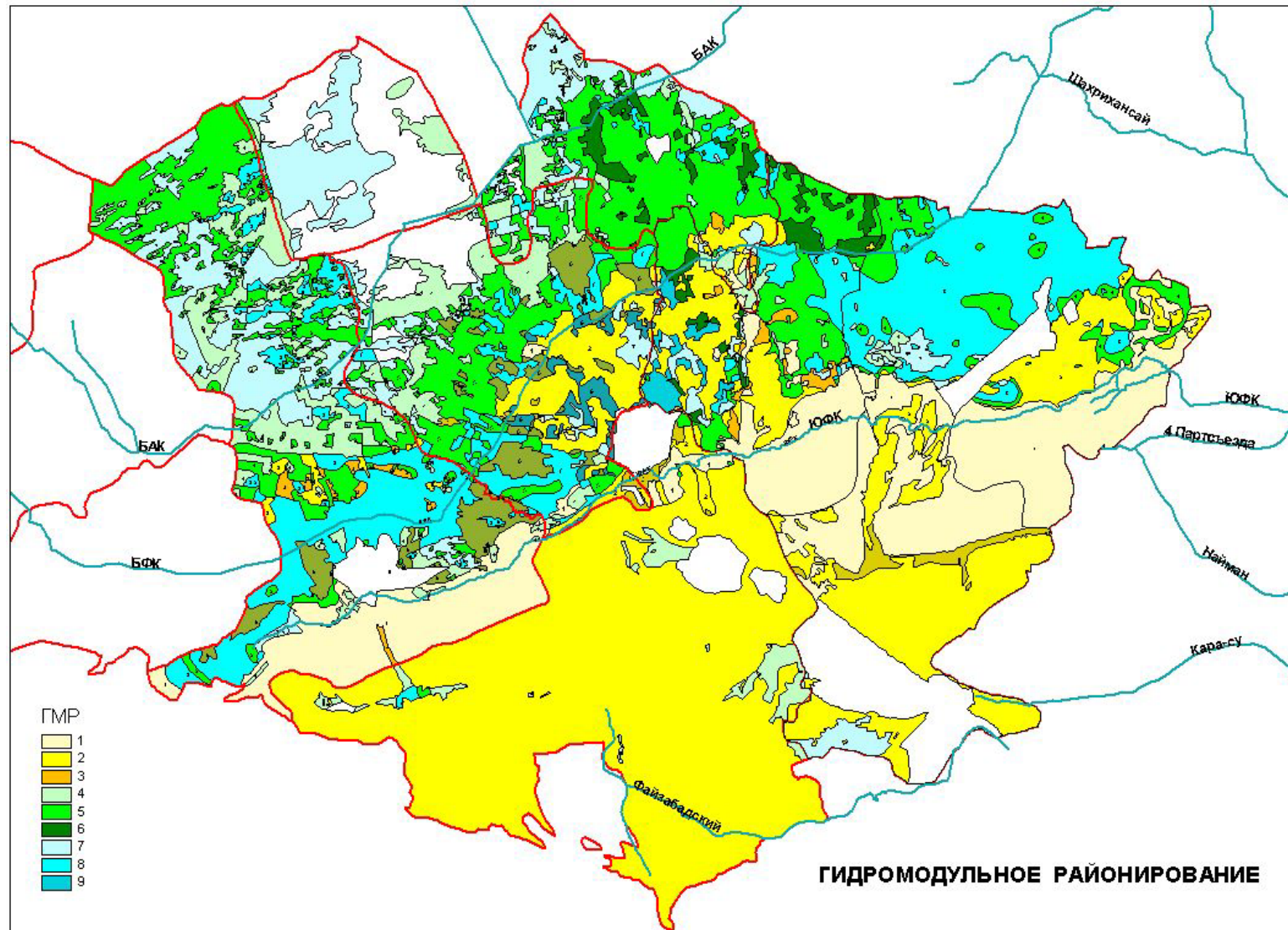
Рис. 7. Гидромодульное районирование
