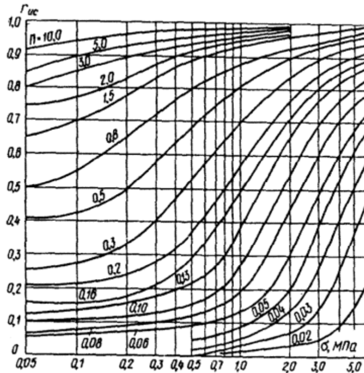
Черт. 1. Номограмма для определения коэффициента парового давления \gamma_{uc}
