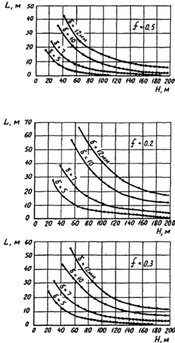
Черт. 1. Зависимость расстояния между горизонтальными швами диафрагмы по высоте L от толщины диафрагмы d , величины коэффициента трения грунта по диафрагме f и высоты диафрагмы H
