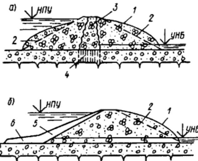
Черт. 7. Виды взрывонабросных плотин
