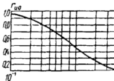
Черт. 3. График зависимости коэффициента порового давления r_{uo} от \sigma_v^o
