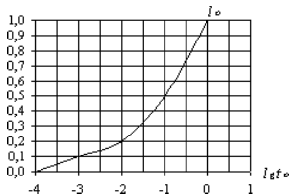
Рис. 2. График для определения величины l_0
