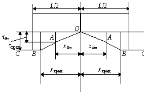
Рисунок. Эпюра касательных напряжений
