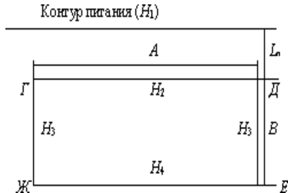
Рис. 1. Схема к расчету водопритоков к одиночной выработке
