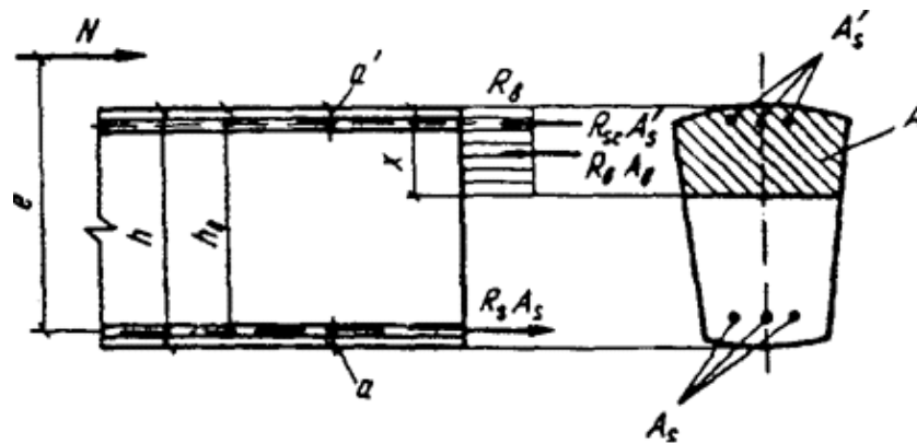
Черт. 3. Схема усилий и эпюр напряжений в сечении, нормальном к продольной оси внецентренно сжатого железобетонного элемента, при расчете его по прочности
