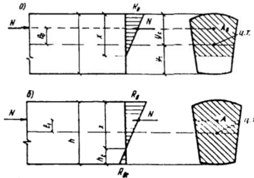
Черт. 1. Схема усилий и эпюра напряжений в сечении, нормальном к продольной оси внецентренно сжатого бетонного элемента
