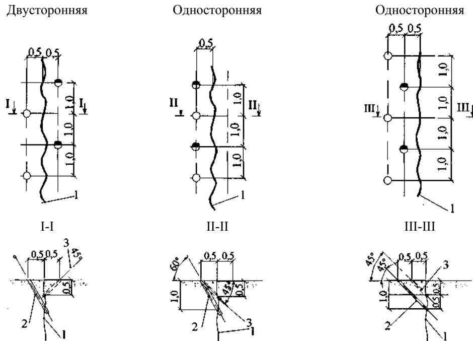
1 - трещина; 2, \circ - скважины I очереди; 3, \bullet - скважины II очереди. Размеры в метрах
