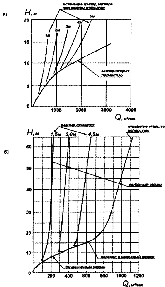
а - безнапорный поверхностный водосброс Вилойских ГЭС-1 и 2; б - глубинный эксплуатационный водосброс Саяно-Шушенской ГЭС
