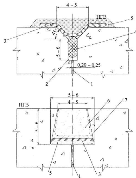
1 - сквозная трещина; 2 - разделка трещины фрезой; 3 - полоса армоэластика; 4 - жгут поризола или чернота; 5 - приклейка полимерным материалом; 6 - цементно-песчаный раствор; 7 - цементно-песчаный раствор с адгезионными добавками Размеры в сантиметрах
