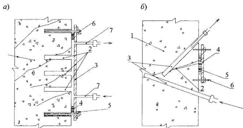
Рисунок Л.3.18 - Принципиальная схема установки для нагнетания цементного раствора
