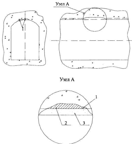
Рисунок Л.3.12 - Тампон-нагнетатель с прижимной плитой
