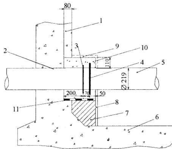
1 - внутренняя сторона стены; 2 - кольцевая ниша; 3 - среднее сборное стальное кольцо; 4 - большое сборное стальное кольцо; 5 - трубопровод; 6 - днище; 7 - опорный фундамент; 8, 9 - опалубочные шины; 10 - изолирующий куб; 11 - прокладка из рубероида. Размеры в сантиметрах
