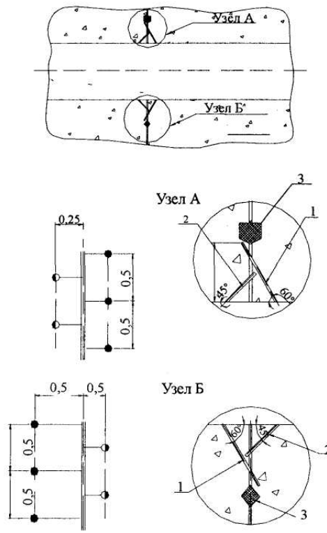
Схема бурения и инъекции: 1, ● - скважины I очереди; 2, ● - скважины II очереди; 3 - битумная шпонка Размеры в метрах
