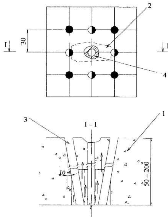
Рисунок Л.3.10 - Тампон-нагнетатель для глубоких скважин
