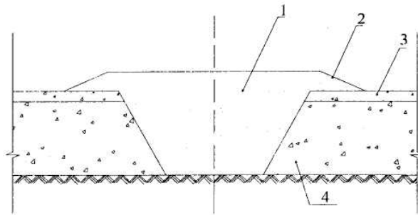
1 - цементно-песчаная пробка; 2 - откос; 3 - бетонная стяжка; 4 - бетонная подготовка пола (днища)
