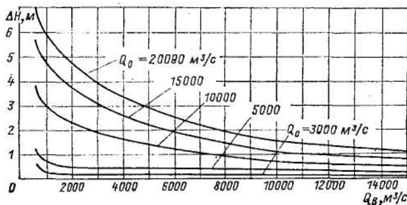
Рисунок И.1.1 - Кривые Q = f(H) в створе Нижегородской ГЭС в зависимости от расхода р. Оки (а) и графики подпора уровня \Delta H при различных расходах Волги Q_B и Оки Q_0 (а)
