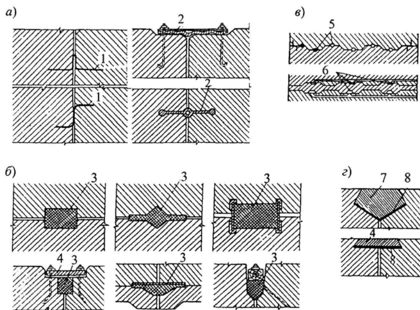
a - диафрагмы из металла, резины и пластических масс; б - шпонки и прокладки из асфальтовых материалов; в - инъекционные (цементация и битумизация) уплотнения; з - брусья и плиты из бетона и железобетона; 1 - металлические листы; 2 - профилированная резина; 3 - асфальтовая мастика; 4 - железобетонная плита; 5 - скважины для цементации; 6 - цементационные клапаны; 7 - железобетонный брус; 8 - асфальтовая гидроизоляционная прокладка
