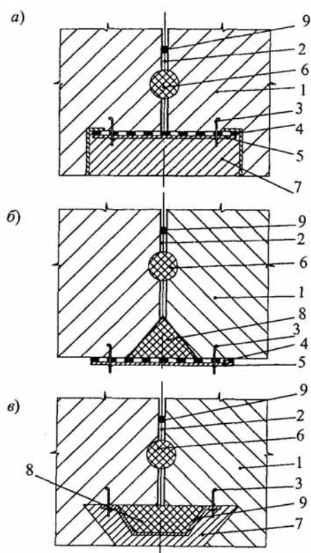
a - внешний компенсатор; б - шпонка на поверхности; в - шпонка внутри; 1 - бетон; 2 - шов; 3 - анкер; 4 - асфальтовый мат; 5 - накладки из листового железа; 6 - дополнительная асфальтовая шпонка; 7 - штрабной бетон; 8 - асфальтовая шпонка; 9 - ограждающая конструкция
