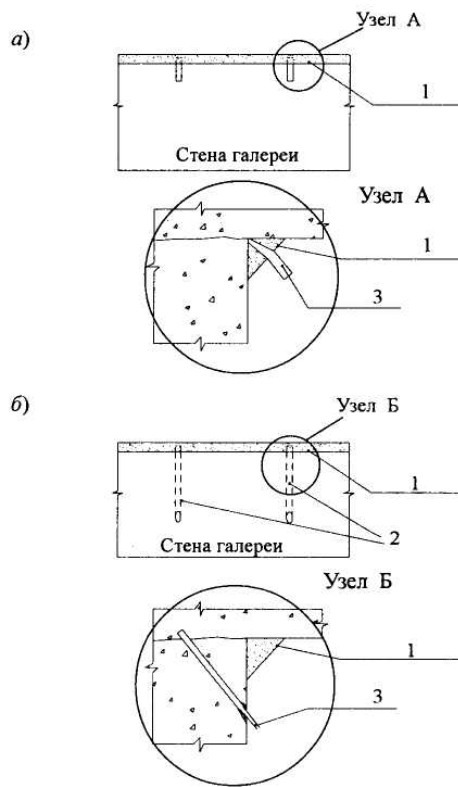
а - вариант без бурения шпуров; б - вариант с бурением шпуров; 1 - цементно-песчаный раствор; 2 - скважина; 3 - патрубков
