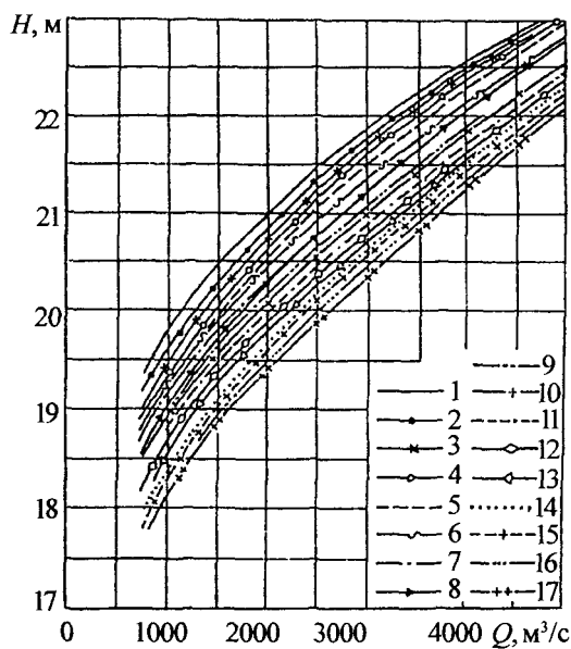
Рис. П1.1. Кривые связи расходов и уровней в нижнем бьефе Новосибирской ГЭС: 1 - проектная; 2 - 1958 г.; 3 - 1959 г.; 4 - 1960 г.; 5 - 1961 г.; 6 - 1962 г.; 7 - 1963 - 1965 гг.; 8 - 1966 г.; 9 - 1967 г.; 10 - 1968 - 1969 гг.; 11 - 1970 г.; 12 - 1971 г.; 13 - 1972 г.; 14 - 1973-1974 гг.; 15 - 1975 г.; 16 - 1975-1978 г.г.; 17 - 1979 - 1980 гг.
