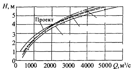
Рис. П1.2. Кривые связи расходов и уровней в нижних бьефах Воткинского (а) и Киевского (б) гидроузлов
