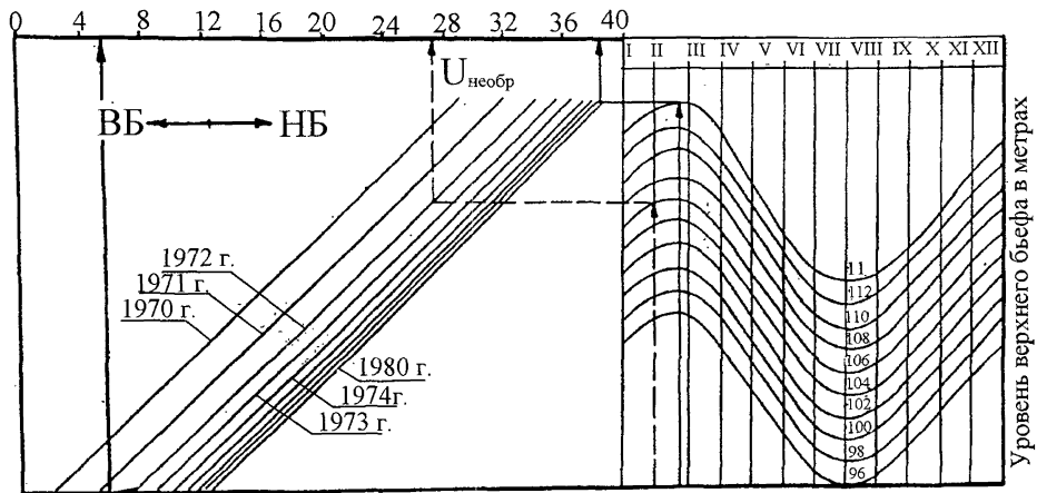
Рис. 1. Номограмма горизонтальных перемещений гребня Красноярской плотины.
