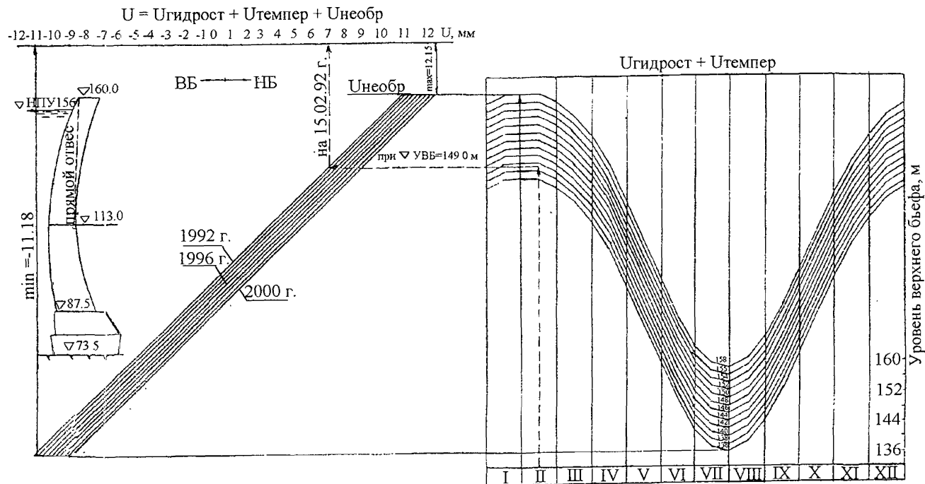
Рис.2. Номограмма горизонтальных перемещений гребня Миатлинской плотины.
