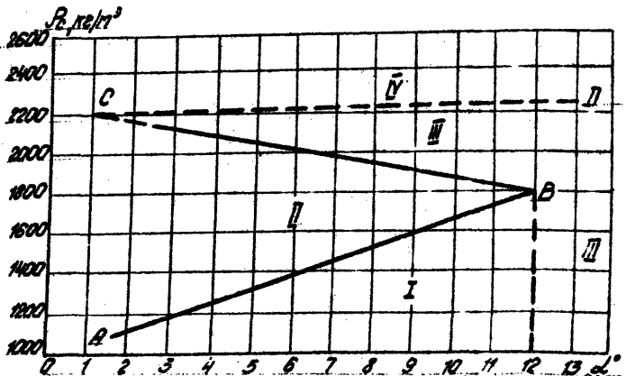
Рис. 2. Зависимость между углом наклона селёного русла, при котором не происходит распад селёной смеси с содержанием частиц размером 2 мм и меньше, составляющим более 35%, и ее плотностью. Обозначения I, II, III, IV те же, что и на рис. 1.
