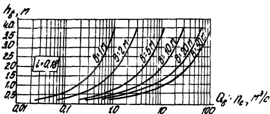
Рис.3 Графики зависимости глубины водного потока h_g от ширины прямоугольного бетонного канала B и величины Q_g \cdot \eta_c при различных уклонах для канала.
