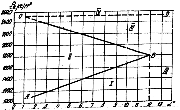
Рис. 1. Зависимость между углом наклона селёного русла, при котором происходит распад; селёной смеси с содержанием частиц размером 2 мм и меньше, составляющим менее 35%, и ее плотностью: I - область обогащения селёной смеси; II - область частичного распада селёной смеси; III - область обогащения селёной смеси; IV - область остановки селё.
