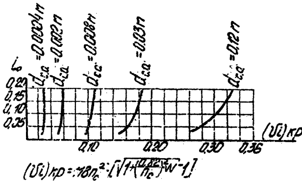
Рис. 4 График зависимости критериальной величины (v \cdot i)_{кр} от уклона i_0 и среднесрежневочного диаметра d_{с.а.} твердой составляющей оседающего потока.
