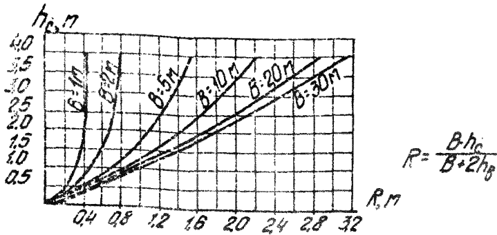
Рис. 7 График зависимости гидравлического радиуса R , и от глубины h_c , м и ширины канала B , м для прямоугольного сечения.
