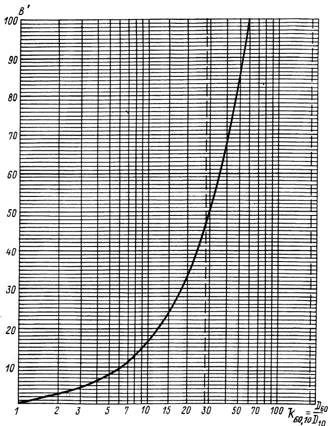
Рис. 24. График B' = f(k_{60,10}) .
