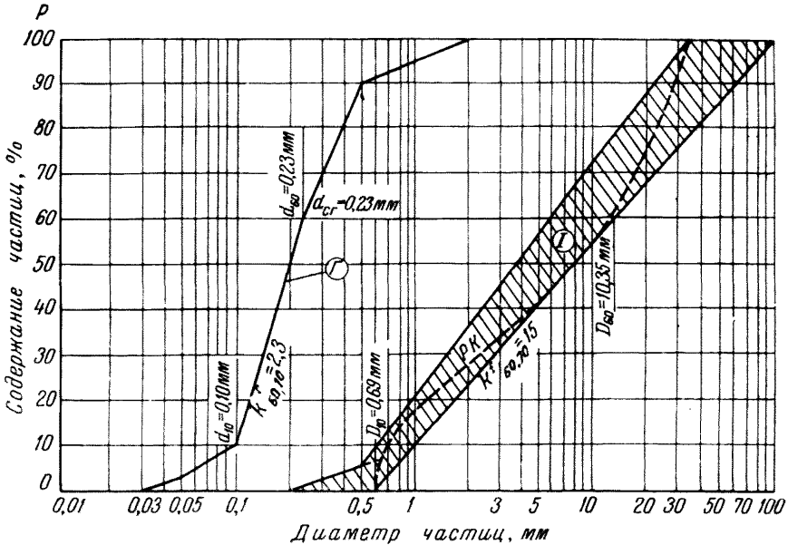
Рис. 10. График запроектованного состава фильтра
