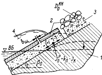
Рис. 34. К проектированию (подбору) фильтровой подготовки под крепления верховых откосов из связного (глинистого) грунта
