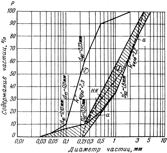
Рис. 18. График допустимого состава фильтра г — грунт тела плотины; I — зона грунтов для фильтра; а — естественный карьерный грунт; НК — несuffузионная кривая, проходящая через D_{10}^I и D_{60}^I карьерного грунта.
