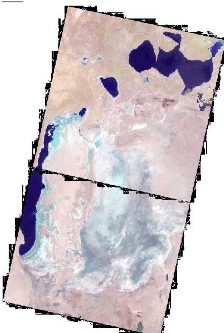
Рисунок 1. Западная и Восточная часть Аральского моря. На основе снимка Landsat 8, 23 Мая 2022.
