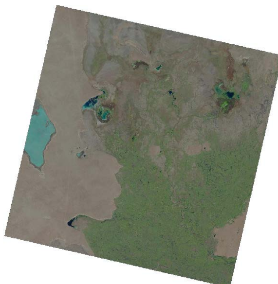
Рис. 2 Приаралье. На основе снимка Landsat 8, 23 Мая 2022.
